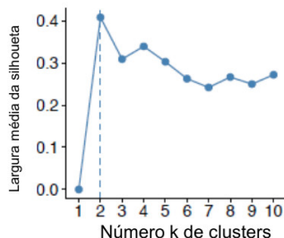
Método Silhouette
