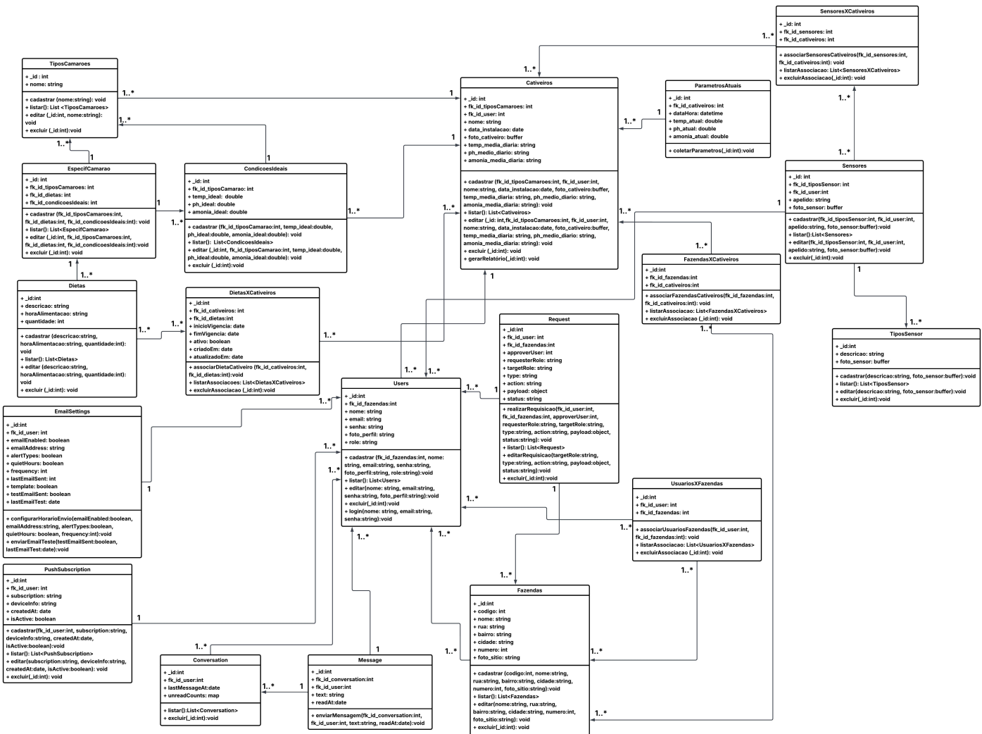
Figura 2 – Diagrama de classe
