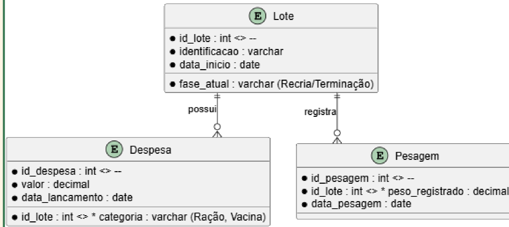
Modelo de Banco de Dados (Entidade-Relacionamento)
