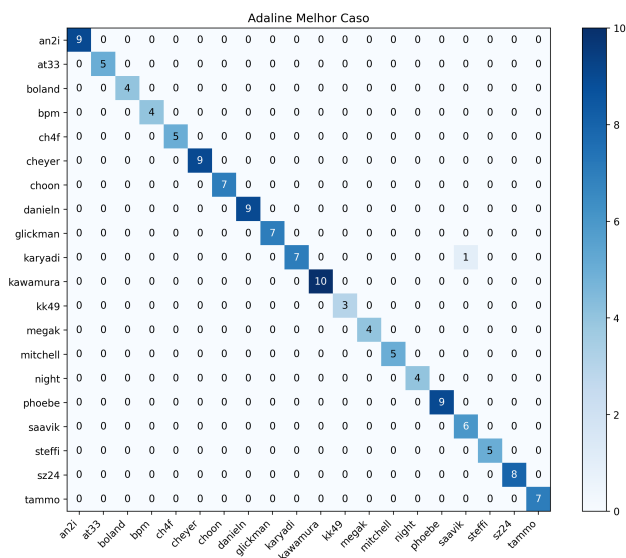
Figura 10. ADALINE: melhor caso.
