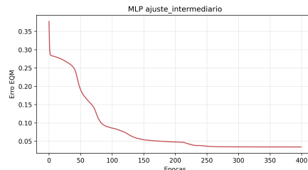
Figura 3. MLP com ajuste intermediário.
