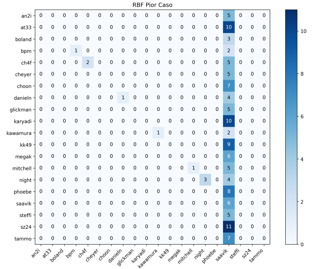
Figura 15. RBF: pior caso.
