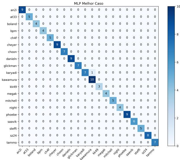
Figura 12. MLP: melhor caso.
