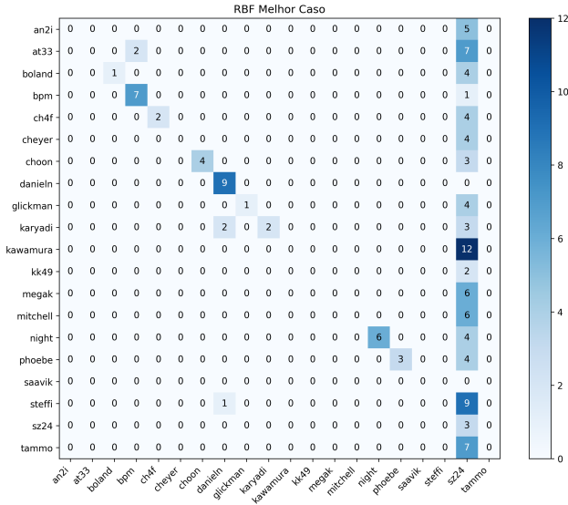
Figura 14. RBF: melhor caso.
