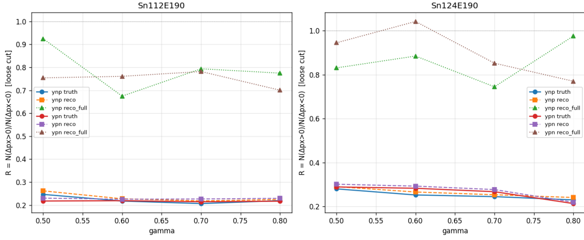
图 3: R_x^{\text{rot}} 随 \gamma (loose cut)。两 panel = 两 target; 圆 = A truth, 方 = B reco mixed, 三角 = C full reco; 线条按 helicity 分。所有 R 值在反应平面 frame。
