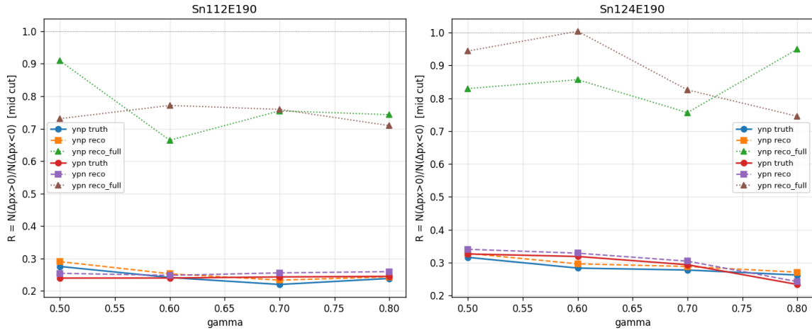
图 4: R_x^{\text{rot}} 随 \gamma (mid cut)。两 panel = 两 target; 圆 = A truth, 方 = B reco mixed, 三角 = C full reco; 线条按 helicity 分。所有 R 值在反应平面 frame。
