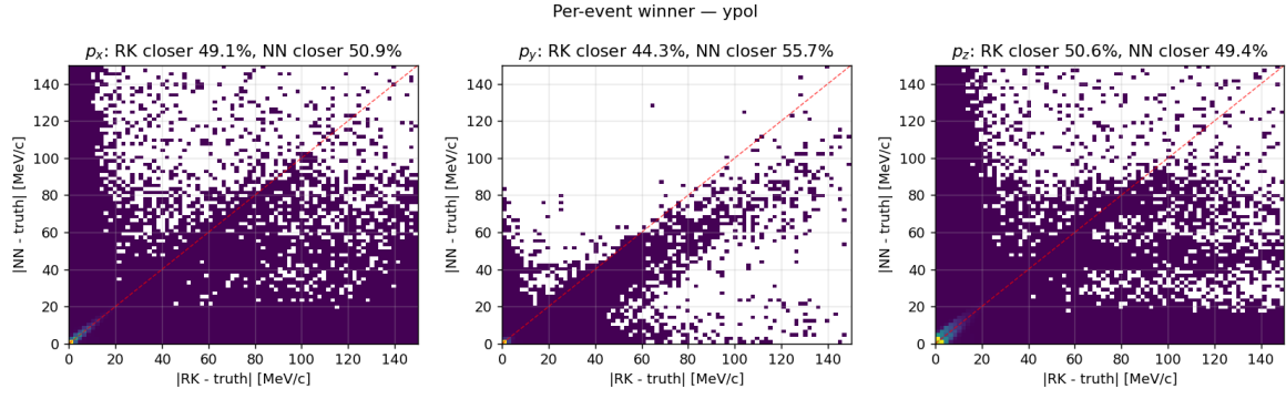
图 5: Per-event winner, ypol。
