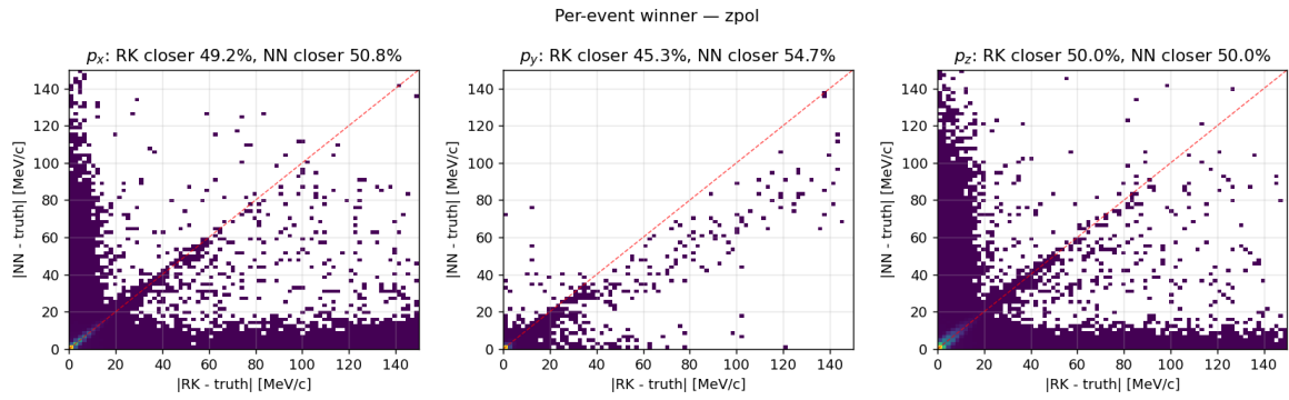
图 7: Per-event winner, zpol。
