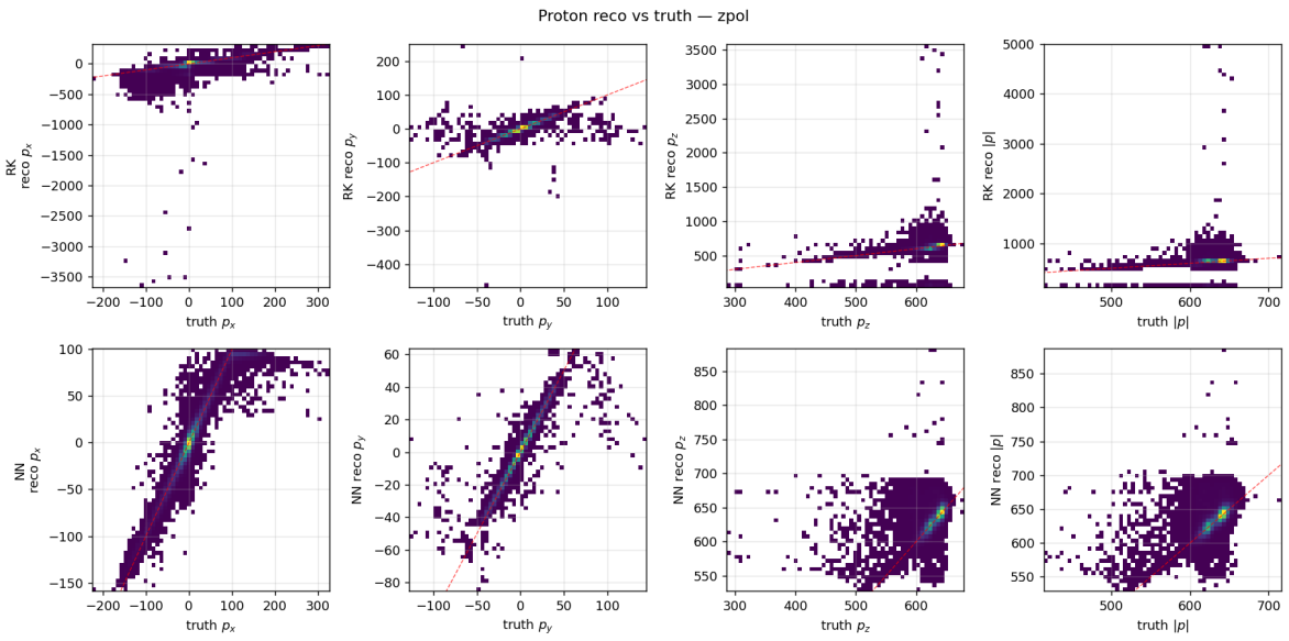
图 4: 质子 reco vs truth 2D 散点, zpol。
