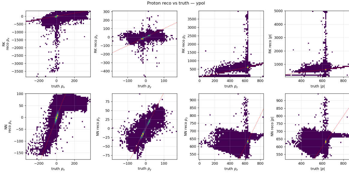
图 2: 质子 reco vs truth 2D 散点, ypol。
