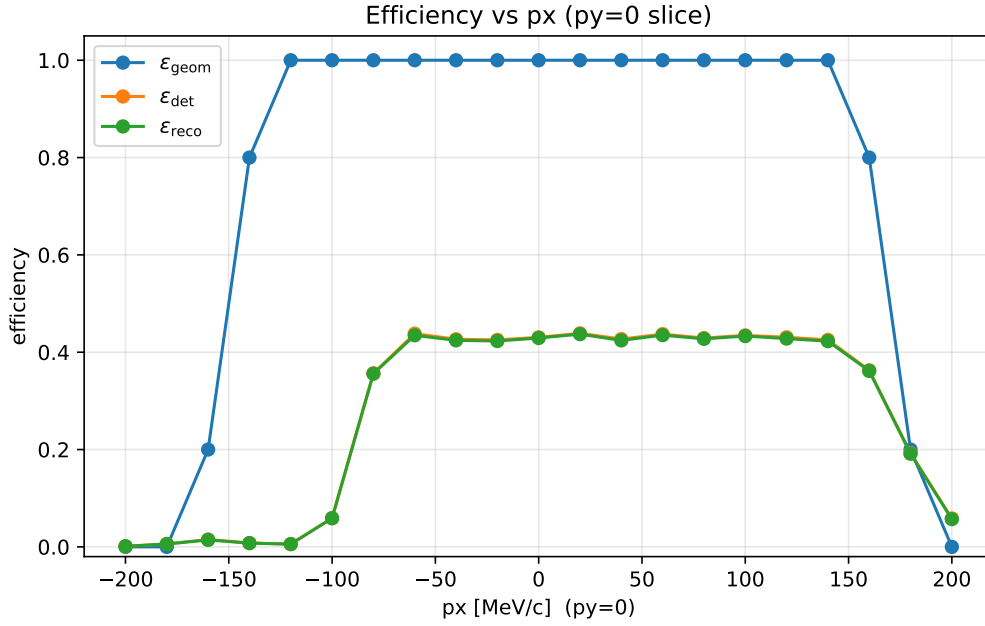
图 5: Fig B2: p_y = 0 切片— \epsilon_{\text{geom}} (蓝)、 \epsilon_{\text{det}} (橙)、 \epsilon_{\text{reco}} (绿) vs p_x 。 \epsilon_{\text{geom}} 在 |p_x| \approx 140 MeV/c 之内为 1.0, 到 |p_x| = 200 MeV/c 降到 0 (两-bin 过渡边)。 \epsilon_{\text{det}} 和 \epsilon_{\text{reco}} 几乎重合在 0.43 平台上, 证明 NEBULA cluster 重建近乎无损。
