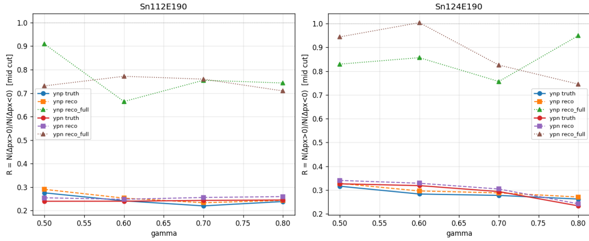
图 2: R_x^{\text{rot}} 随 \gamma (mid cut)。两 panel = 两 target; 圆 = A truth, 方 = B reco mixed, 三角 = C full reco; 线条按 helicity 分。所有 R 值在反应平面 frame。
