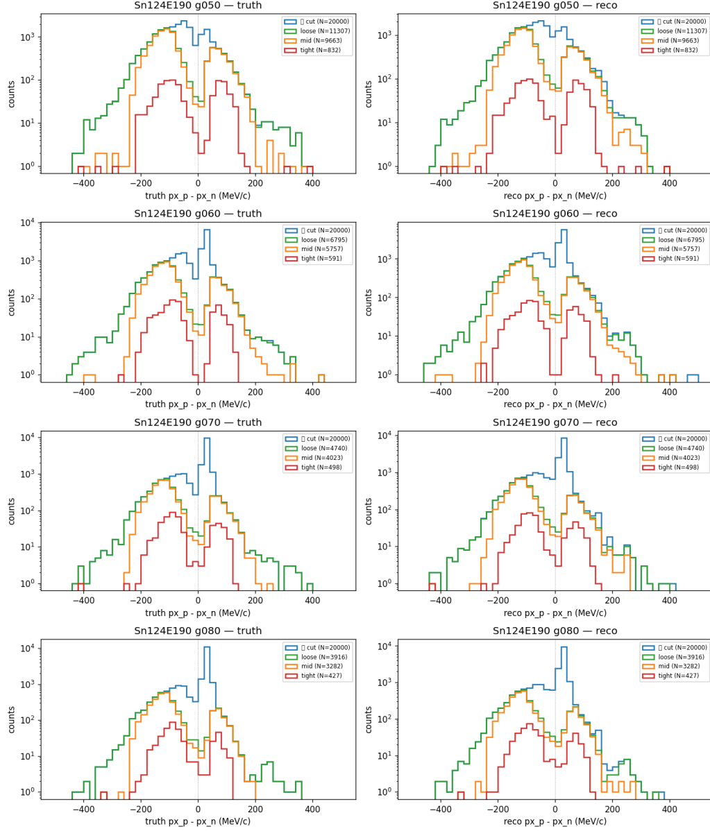
图 11: \Delta p_x^{\text{rot}} 在四 cut 下的叠加 (Sn124E190)。4 行 = 4 gammas, 列 = truth (A) / reco mixed (B)。蓝 = 无 cut, 绿 = loose, 橙 = mid, 红 = tight。
