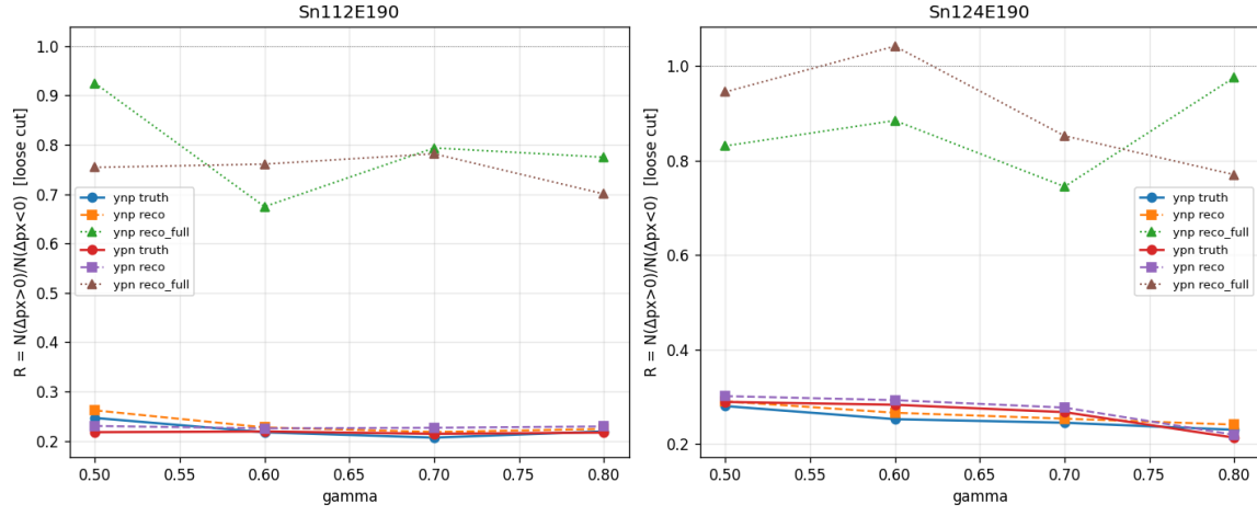
图 1: R_x^{\text{rot}} 随 \gamma (loose cut)。两 panel = 两 target; 圆 = A truth, 方 = B reco mixed, 三角 = C full reco; 线条按 helicity 分。所有 R 值在反应平面 frame。
