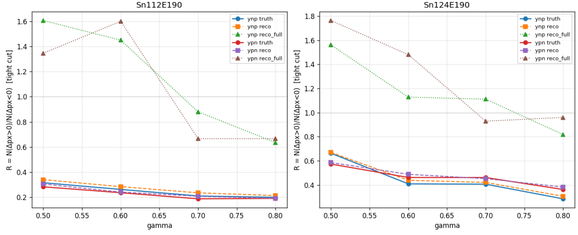
图 3: R_x^{\text{rot}} 随 \gamma (tight cut)。两 panel = 两 target; 圆 = A truth, 方 = B reco mixed, 三角 = C full reco; 线条按 helicity 分。所有 R 值在反应平面 frame。
