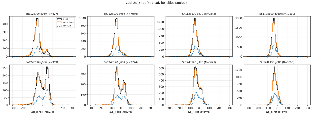
图 12: zpol \Delta p_x^{\text{rot}} 分布 (mid cut).
