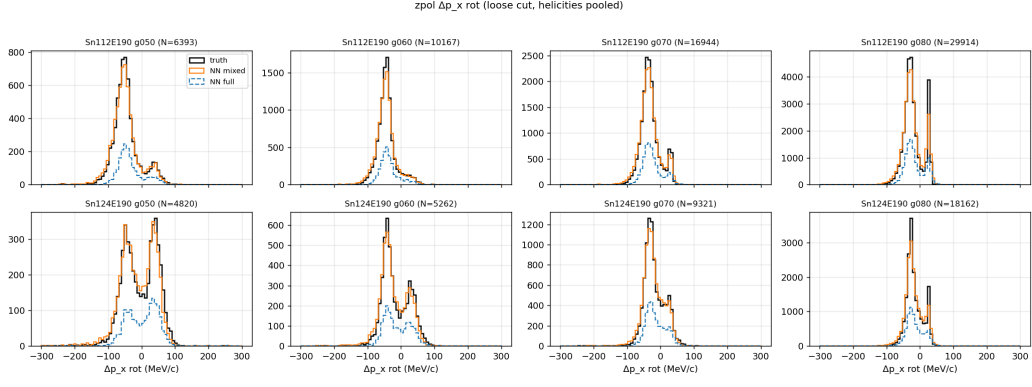
图 11: zpol \Delta p_x^{\text{rot}} 分布 (loose cut).
