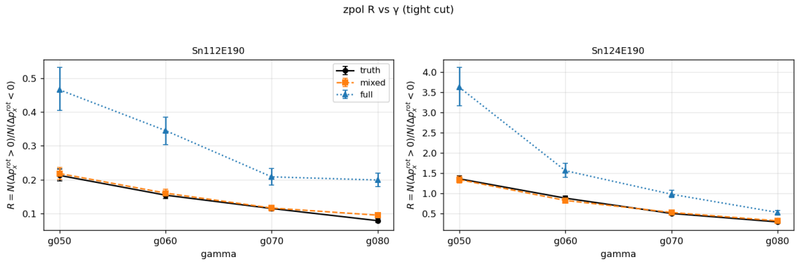
图 10: zpol R_x^{\text{rot}} vs gamma (tight cut).
