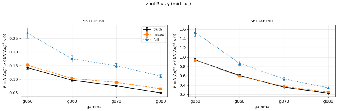
图 9: zpol R_x^{\text{rot}} vs gamma (mid cut).
