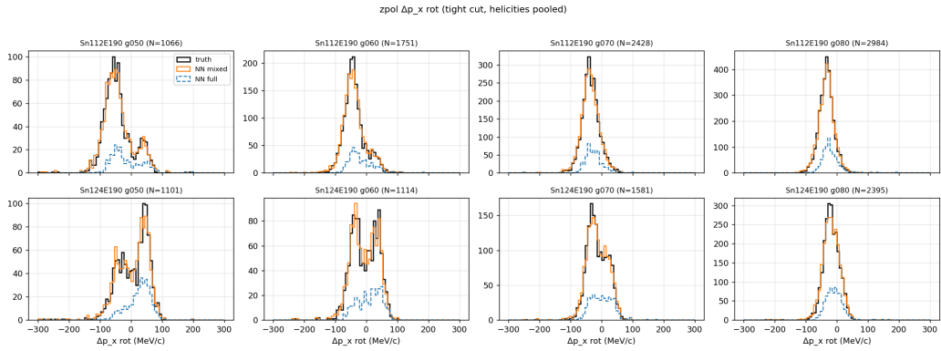
图 13: zpol \Delta p_x^{\text{rot}} 分布 (tight cut).
