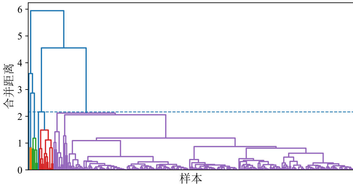
baran · 数据集2 · 树状图 ( k*=5 )
