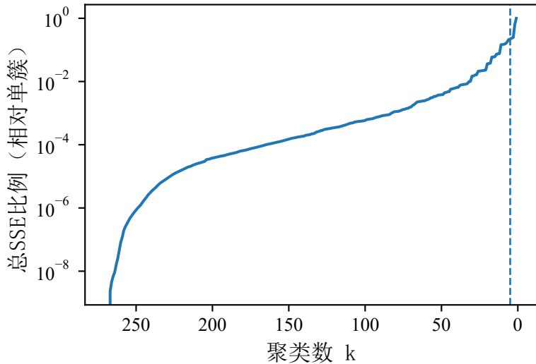
baran · 数据集2 · SSE收敛
