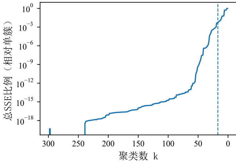
baran · 数据集5 · SSE收敛
