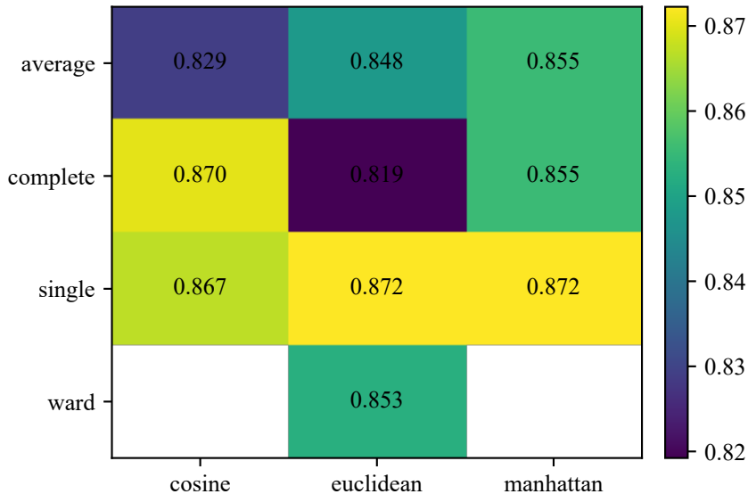
baran • 数据集5 • 配置最佳得分
