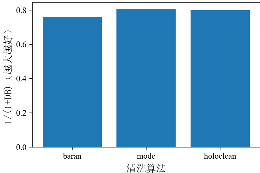
数据集 2 • 1/(1+DB) (越大越好)
