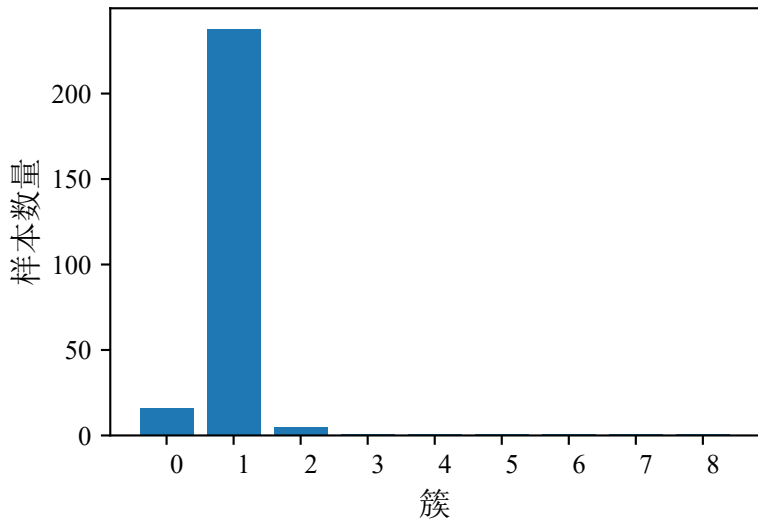
holoclean · 数据集2 · 簇大小
