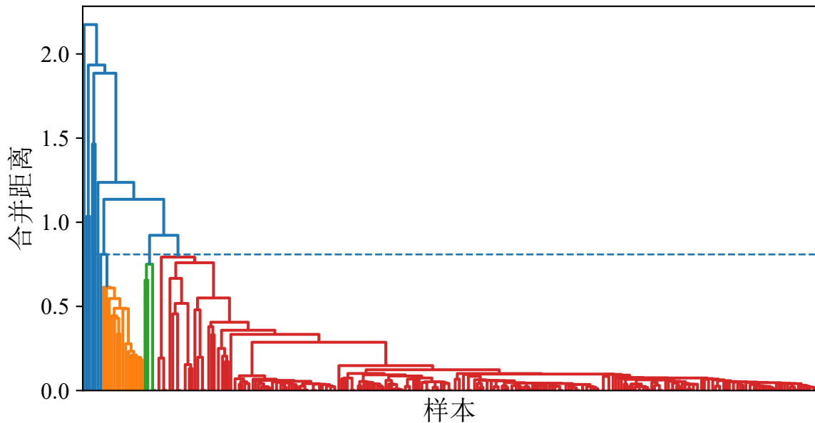
holoclean · 数据集2 · 树状图 ( k^*=9 )
