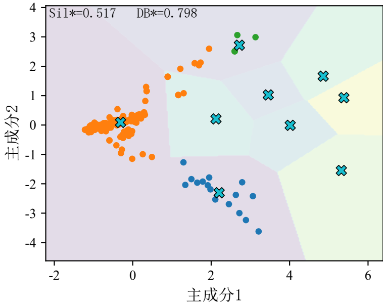
holoclean • 数据集2
