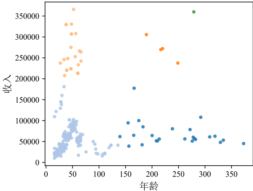
聚类散点 • holoclean • 数据集5
