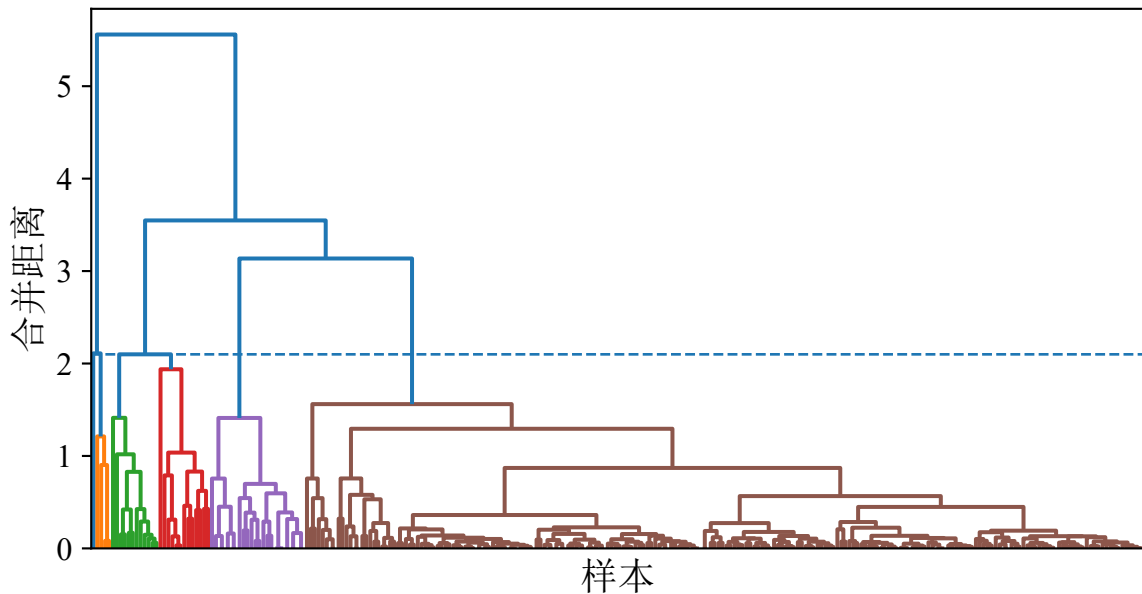
holoclean · 数据集5 · 树状图 ( k*=5 )
