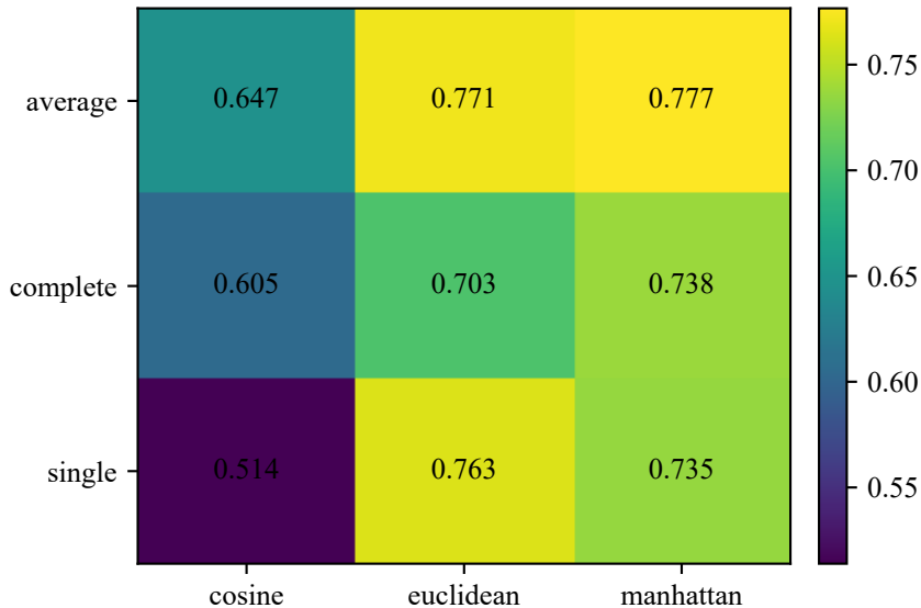
holoclean · 数据集5 · 配置最佳得分
