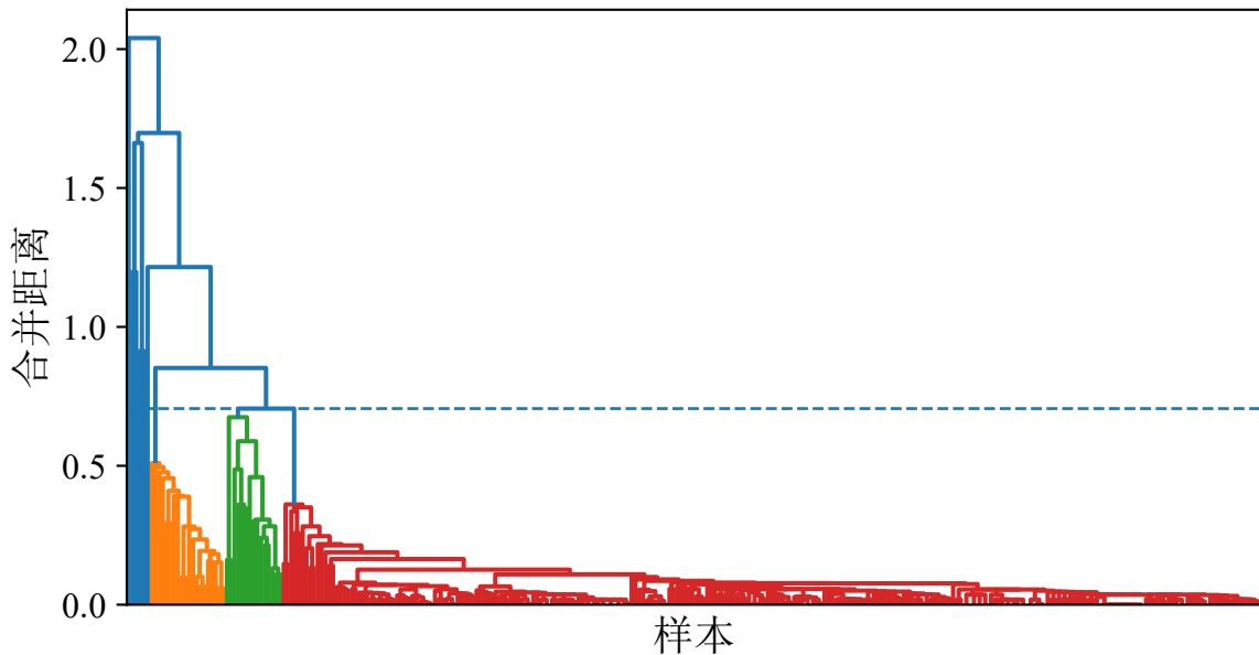
mode · 数据集2 · 树状图 ( k*=8 )
