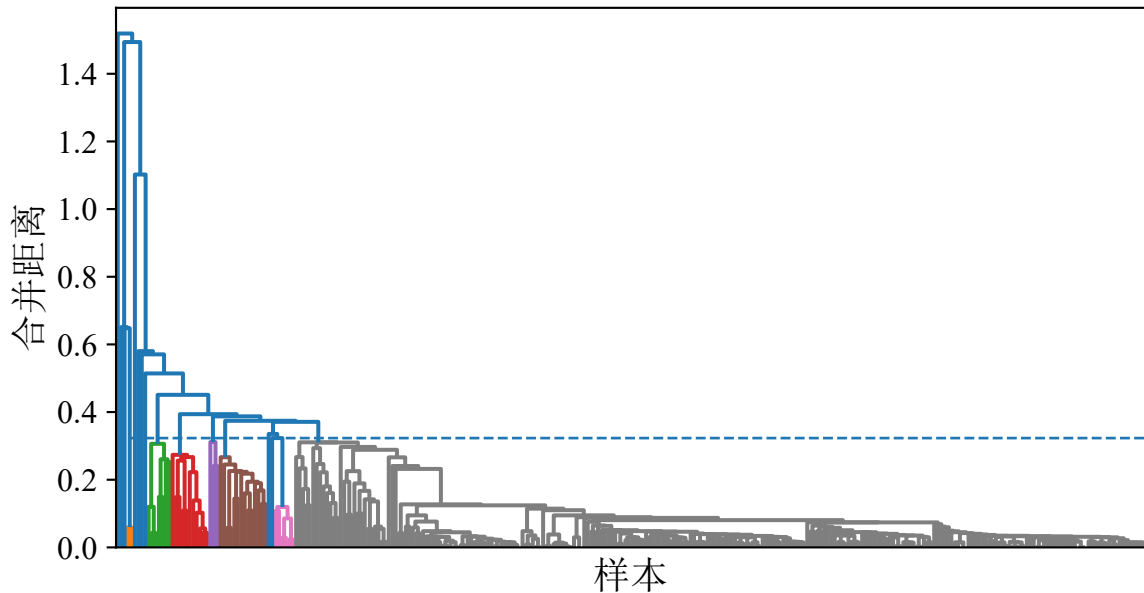
mode • 数据集5 • 树状图 ( k^*=15 )
