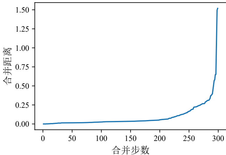
mode · 数据集5 · 合并距离
