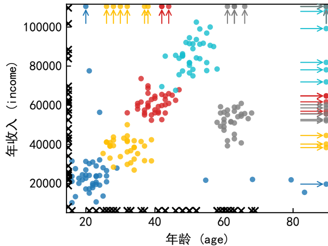
脏数据集：缺失率：15% 异常率：10% 总错误率：25%
