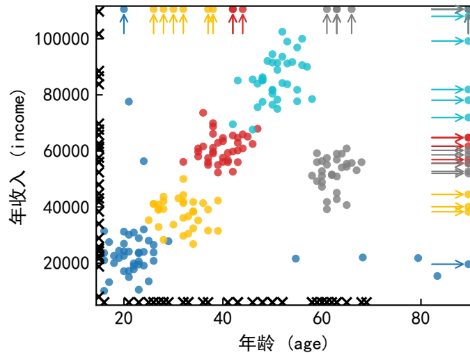
使用boostclean清洗后数据集
