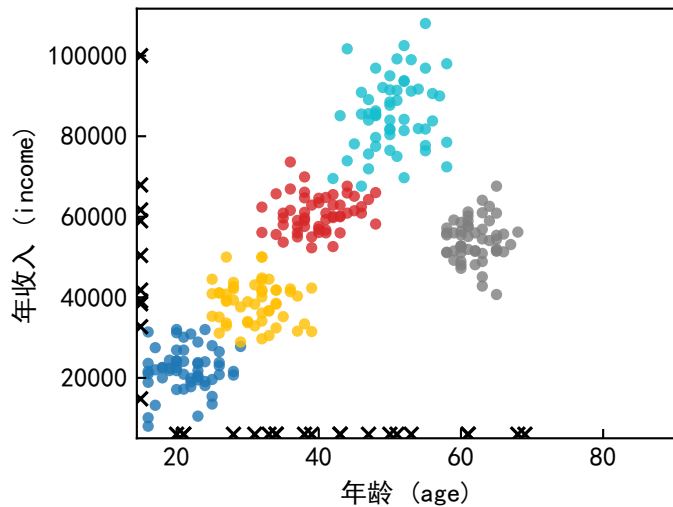
脏数据集：缺失率：5% 异常率：0% 总错误率：5%
