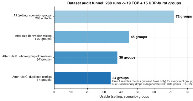
图 2: 数据审计漏斗: 72 个 (设置, 场景) 组合经规则 B (修订混用与整组旧修订)、规则 C (重复配置) 过滤后保留 34 个组合; 规则 A 重写全部保留组合的指标定义, 规则 D 另行排除 4 个退化 BBR 数据点
