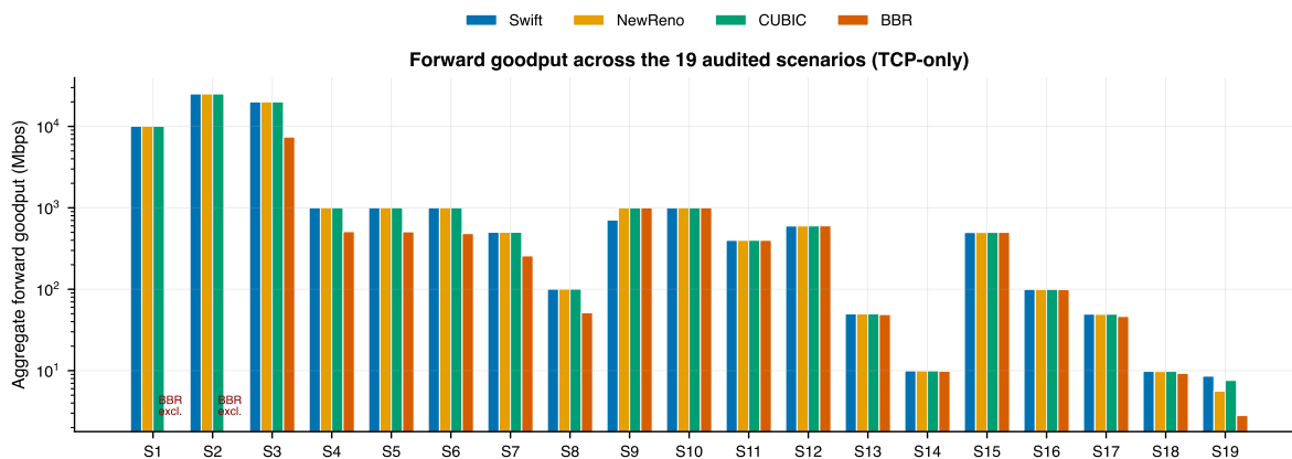
图 3: 19 个审计后场景的聚合前向吞吐量（对数坐标）。S1、S2 的 BBR 数据点按规则 D 排除
