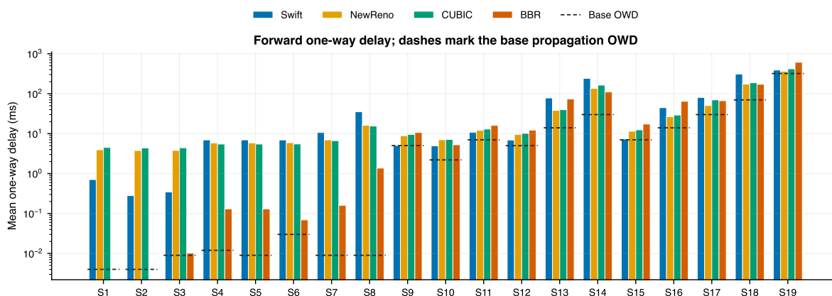
图 4: 19 个场景的平均单向前向延迟（对数坐标）。黑色短划线为各场景的基线单向传播时延，柱顶与短划线的距离即排队分量
