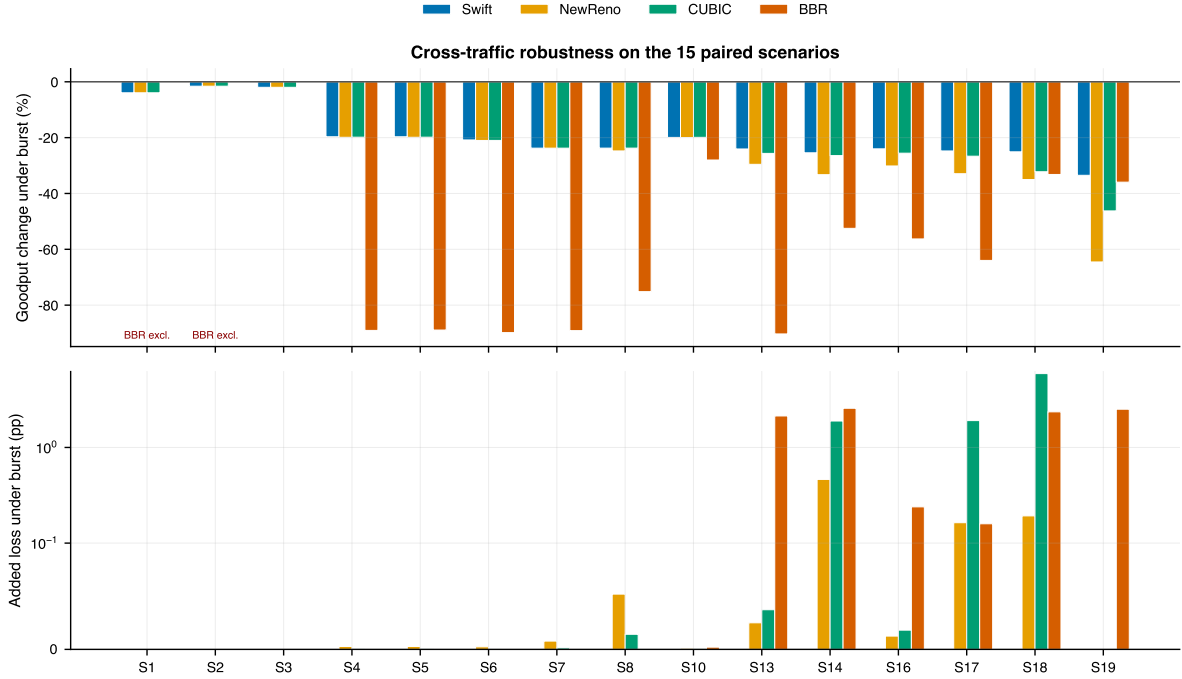
图 5: 15 个配对场景的跨流量鲁棒性: UDP 突发引起的吞吐量变化 (上) 与新增丢包 (下, 符号对数坐标)。Swift 无新增丢包, 故下半幅不存在对应柱体; S1、S2 的 BBR 按规则 D 排除
