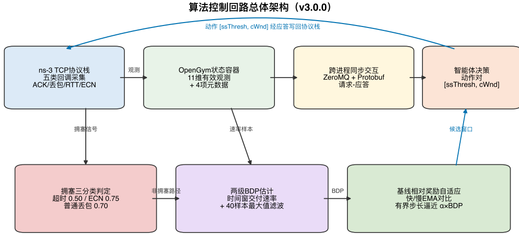
图 1: Swift 控制回路总体架构: 协议栈回调采集的观测经 OpenGym 容器与 ZeroMQ 同步信道送入智能体, 智能体内部依次执行拥塞三分类判定、两级 BDP 估计与基线相对奖励自适应, 动作对经应答写回协议栈
