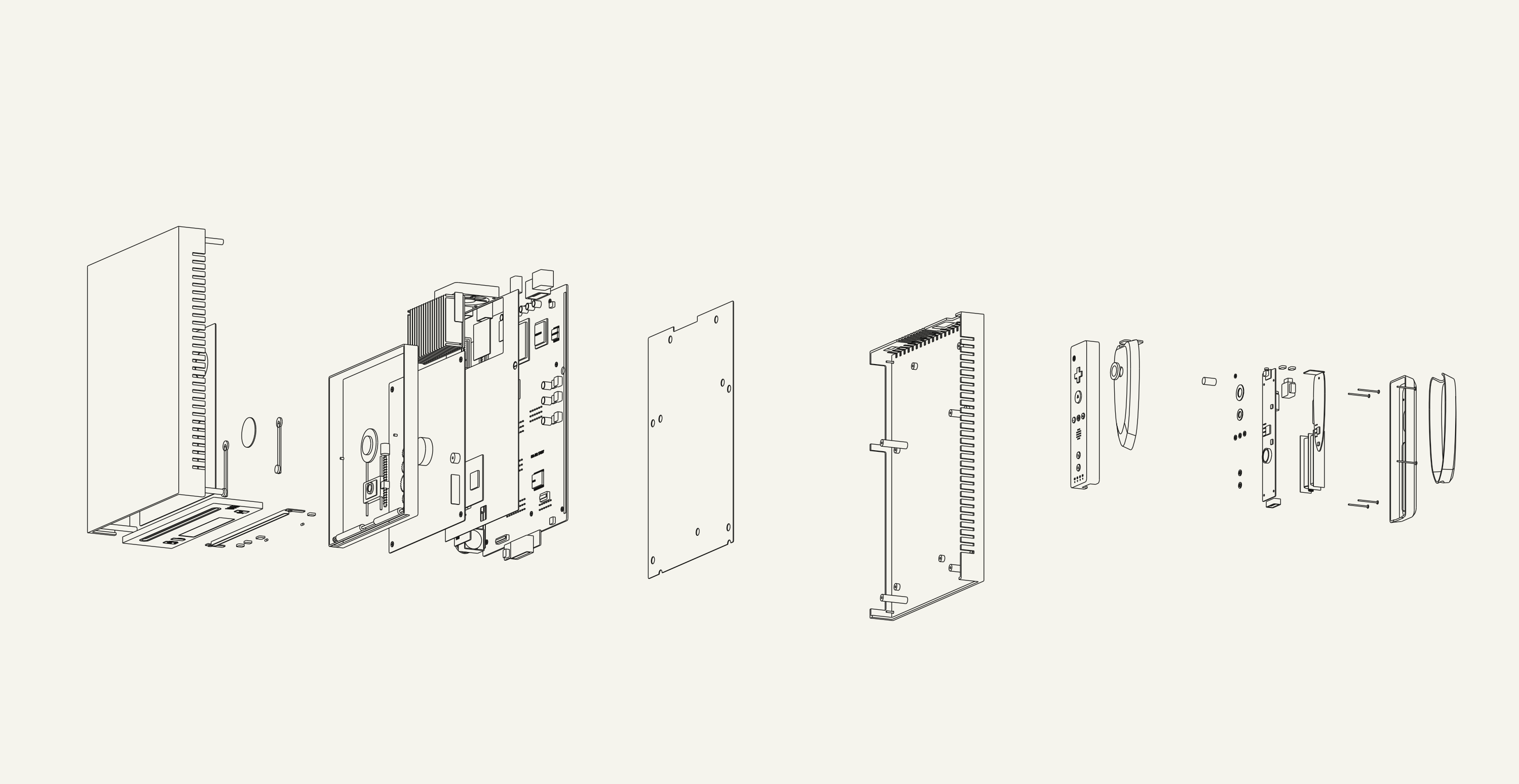
主机壳体、光驱、板件与支承 · 0.339:1
