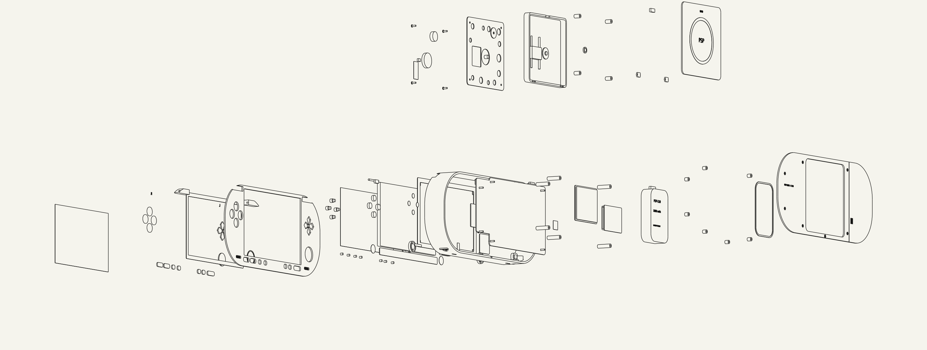
完整主机 · 展示偏移 · 0.471:1
