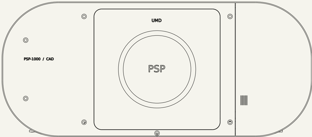
后壳、电池盖与 UMD 门 · 0.979:1
