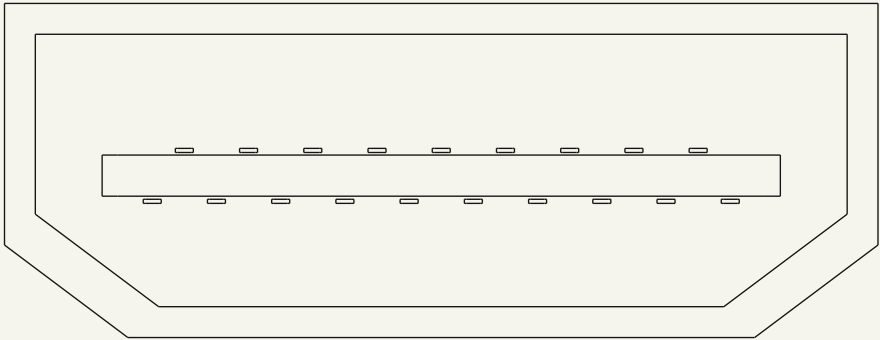
十九接点 HDMI Type A · 6.797:1
