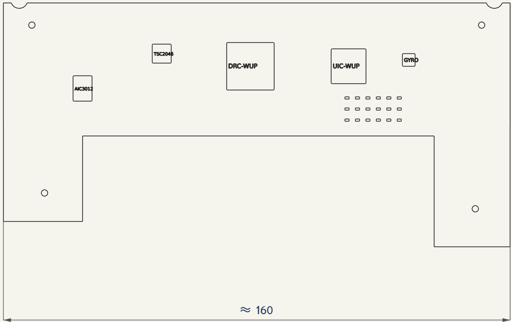
主控制板与主要器件 · 0.852:1
