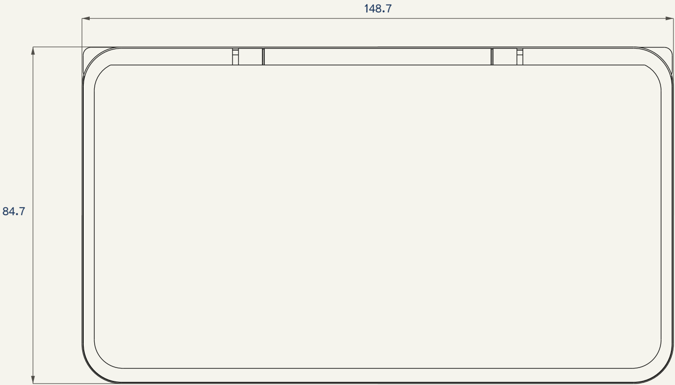
闭合上视 · 1.050:1
