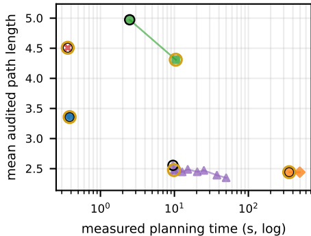
● RBF ◆ IRIS-NP+GCS ■ PRM × RRTConnect ▲ BIT*
