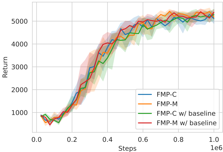
Ant-v4
