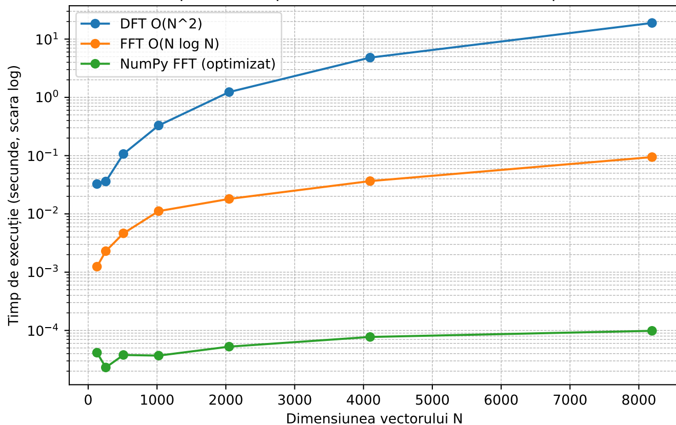
Compararea timpilor de executie: DFT vs FFT vs np.fft.fft
