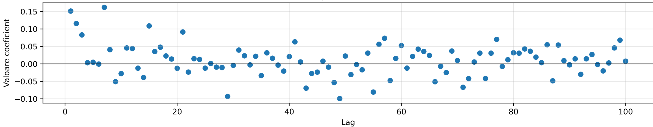
Coeficienți AR Greedy (sparse) max_features=33
