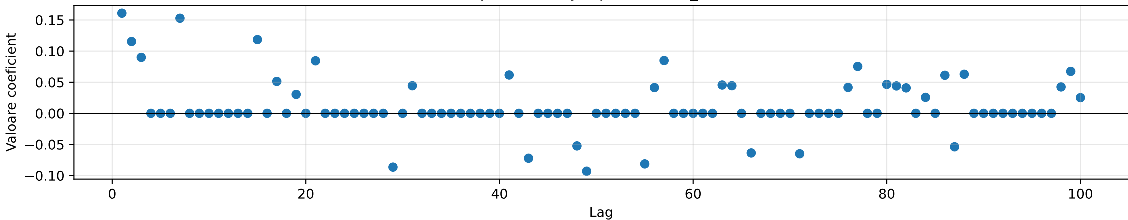
Coeficienți AR LASSO (L1) l=10
