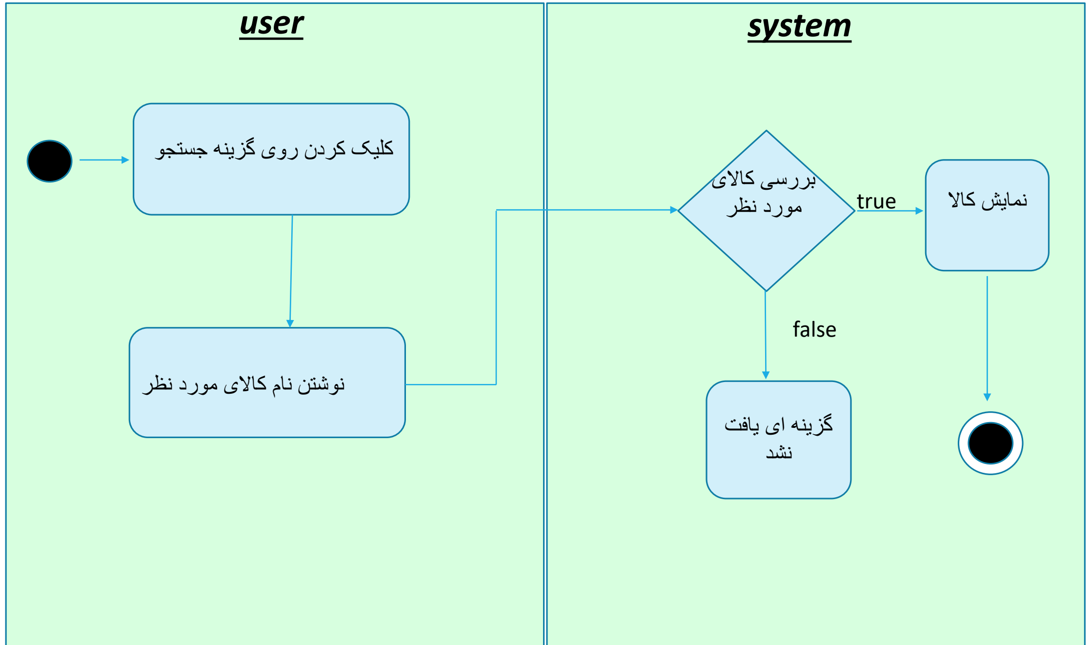
swimlane Diagram نحوه جستجو کردن در سایت:
