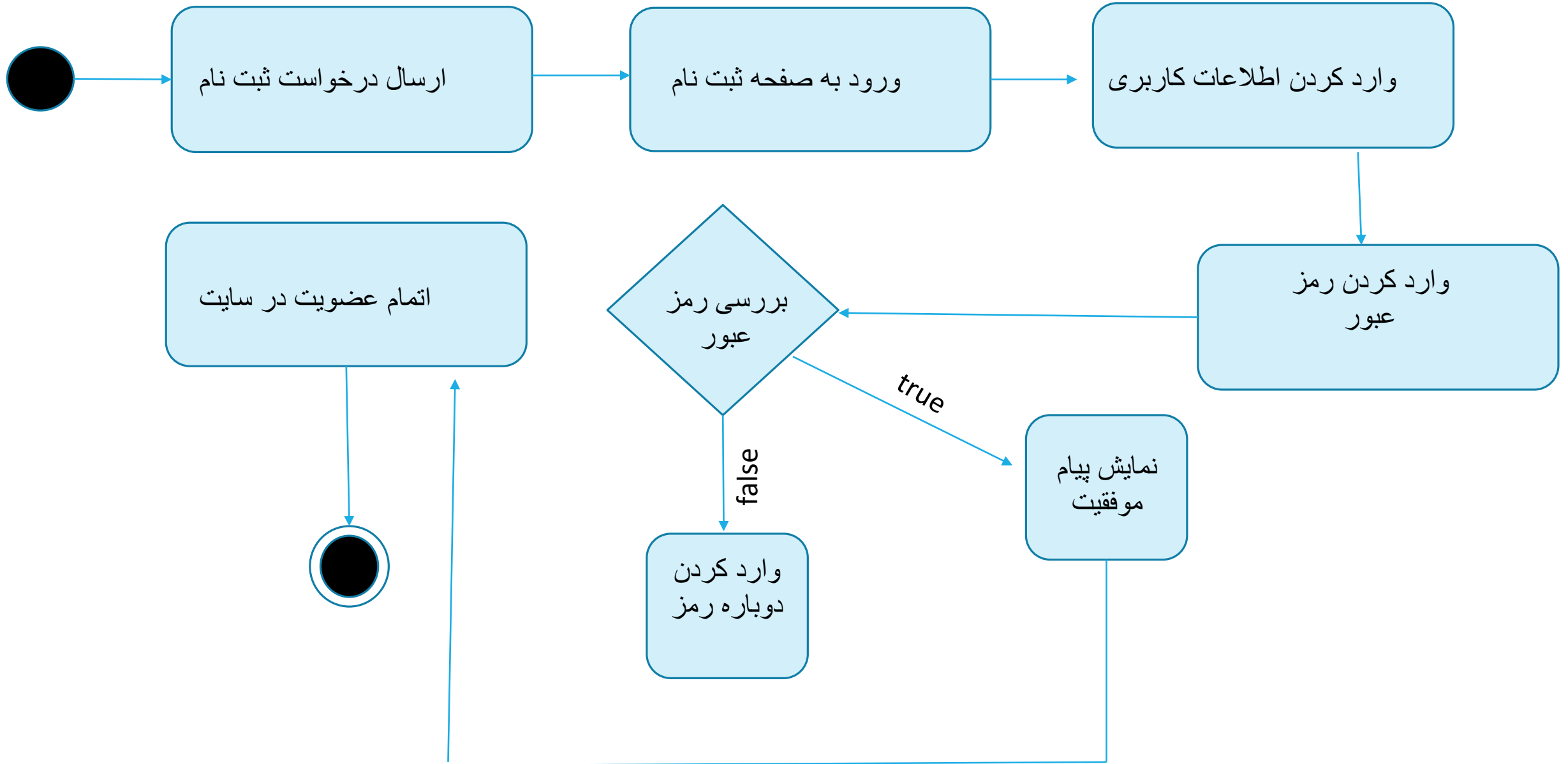
activity diagram نحوه عضویت در سایت:
