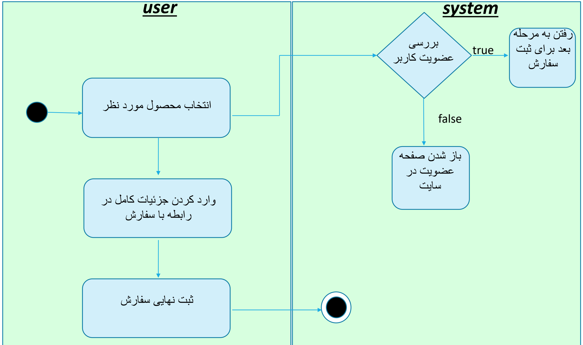
swimlane Diagram نحوه ثبت سفارش در سایت:
