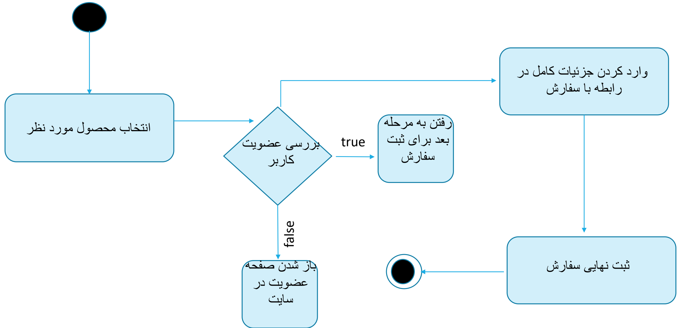
activity diagram نحوه ثبت سفارش در سایت:
