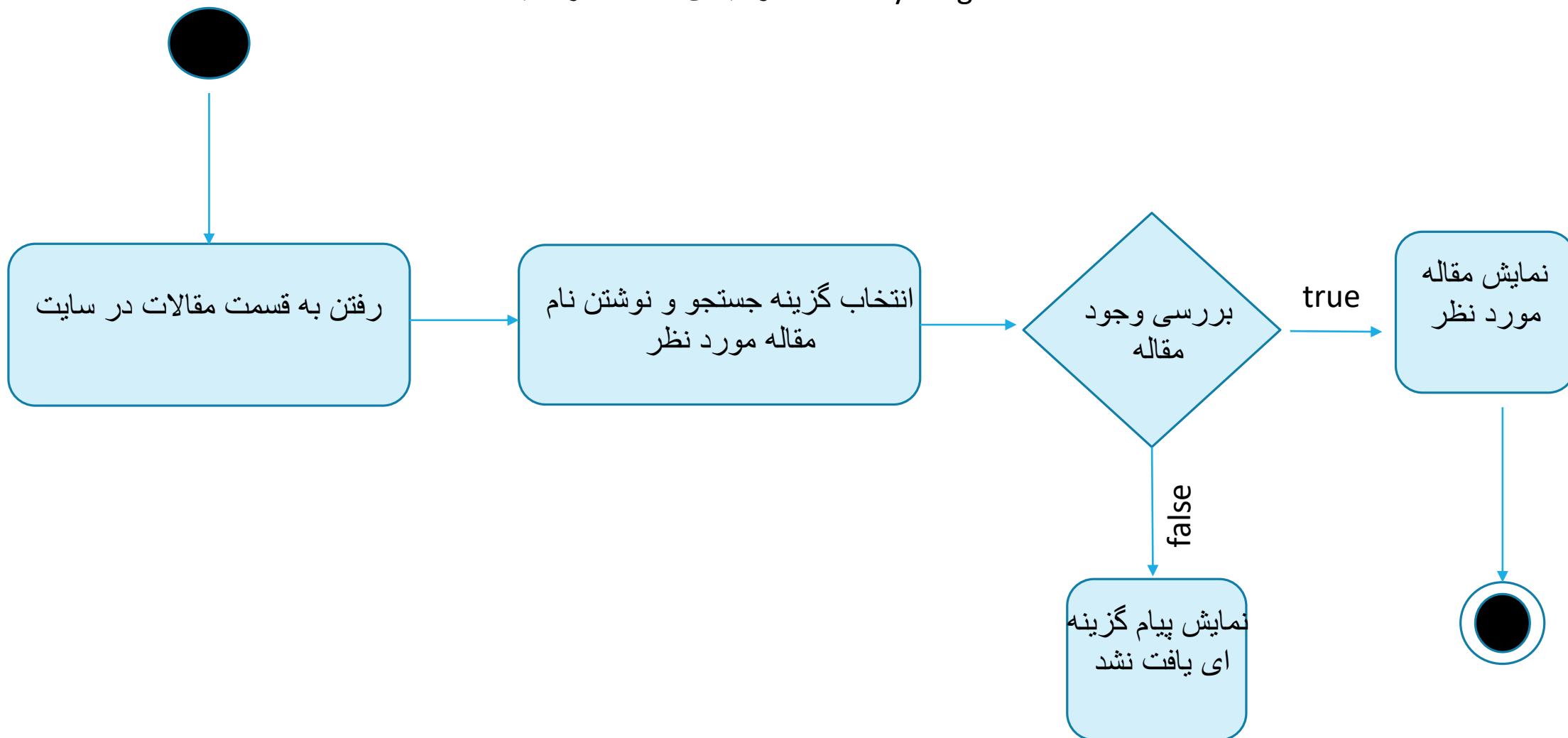
activity diagram نحوه یافتن مقالات در سایت:
