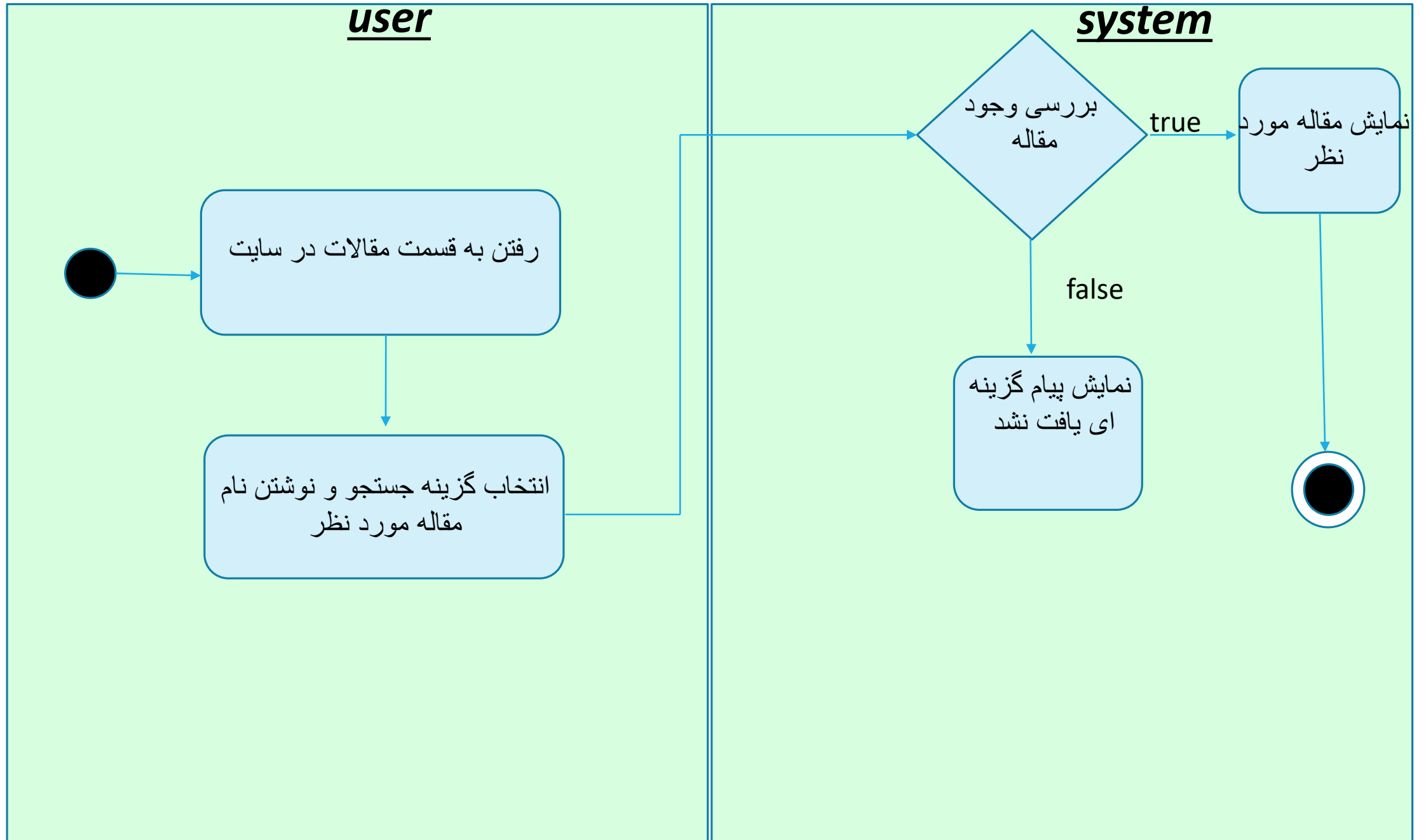
swimlane Diagram نحوه یافتن مقالات در سایت:
