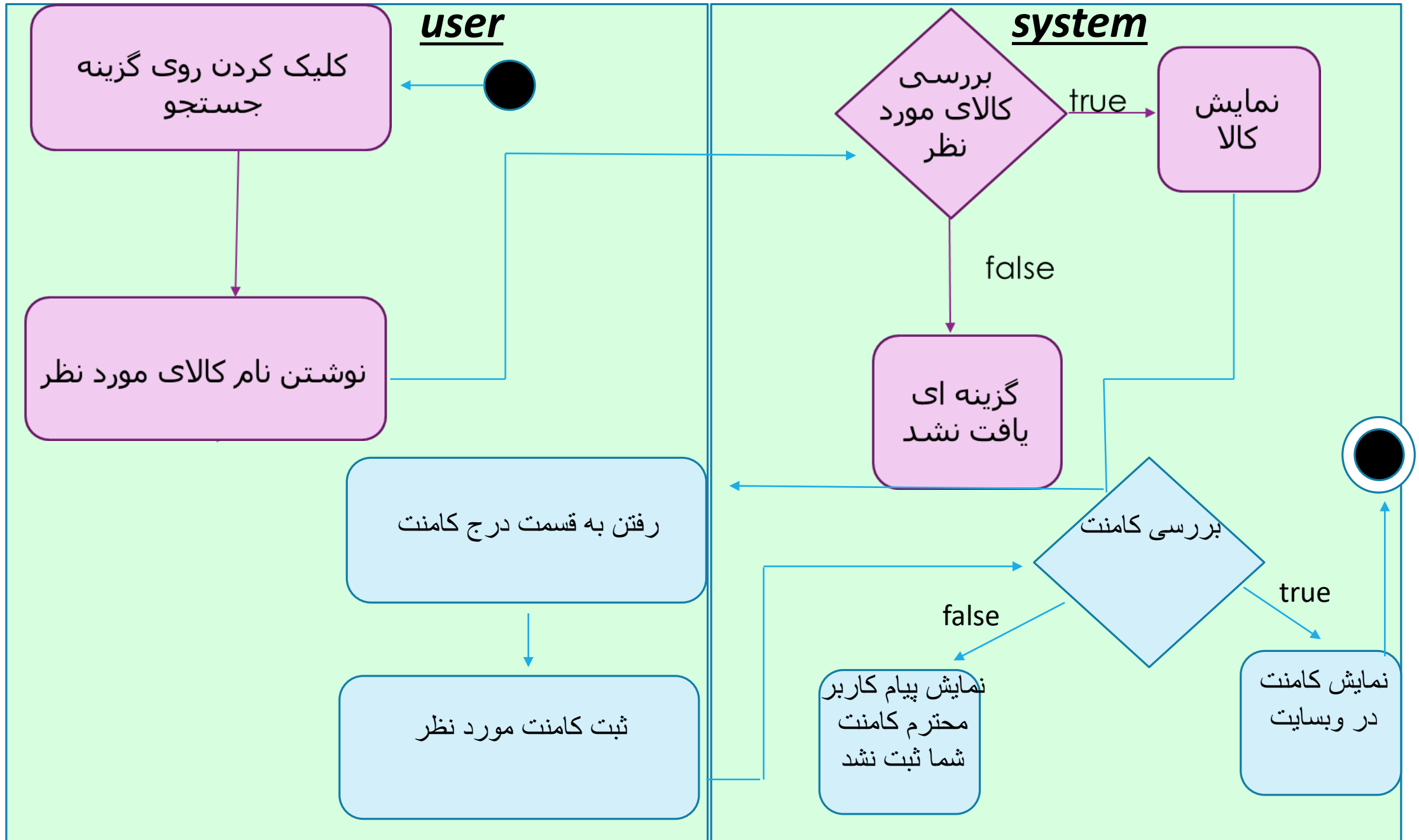
swimlane Diagram نحوه درج کامنت در سایت:
