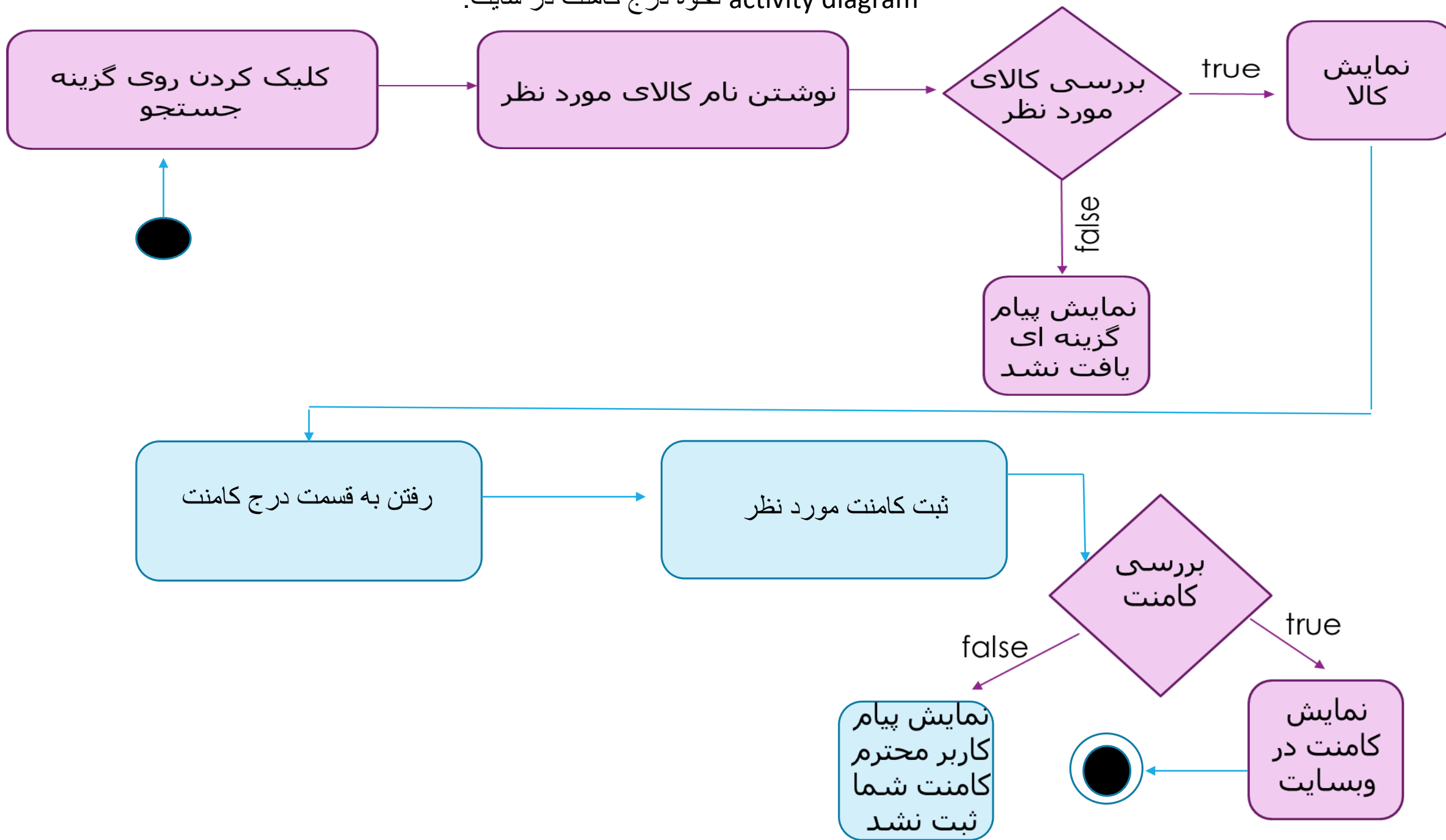
activity diagram نحوه درج کامنت در سایت:
