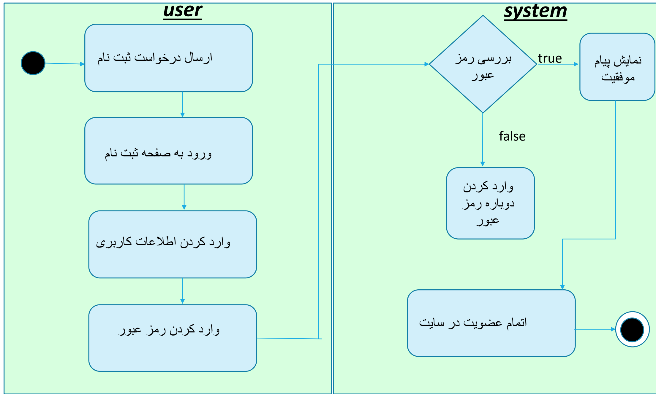
swimlane Diagram نحوه عضویت در سایت:
