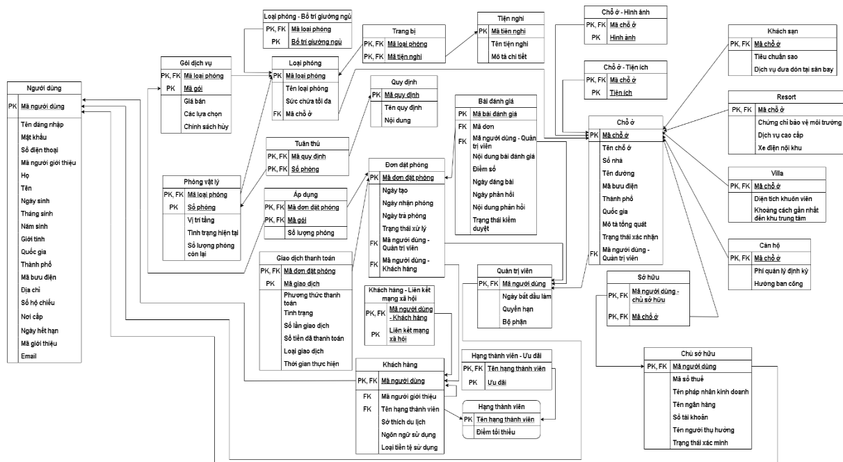
Hình 4.1 – Lược đồ ánh xạ từ EERD hệ thống đặt phòng khách sạn
