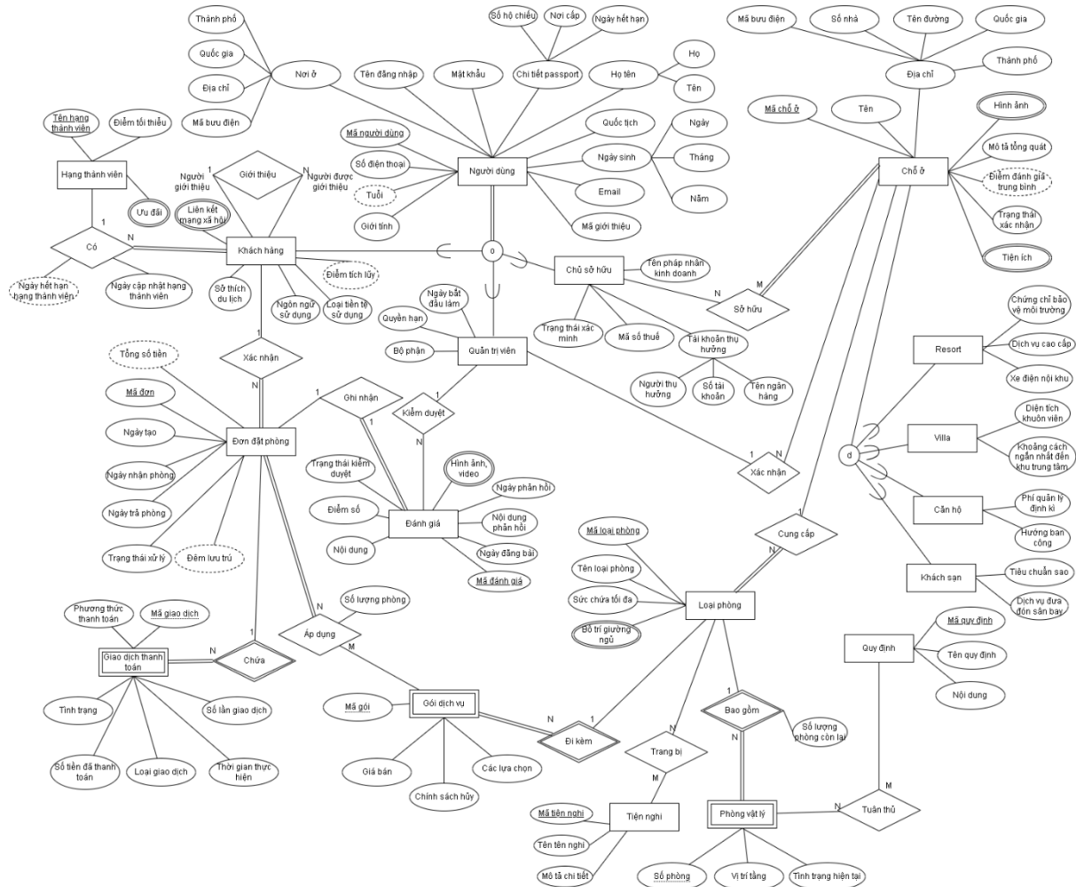
Hình 3.1 – Mô hình thực thể mối liên kết cho hệ thống đặt phòng khách sạn
