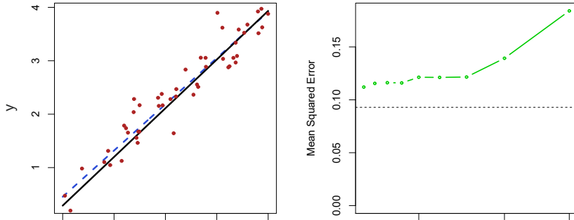
HÌNH 3.3. Khảo sát tiếp dataset trong Hình 3.17. Trái: Đường xanh đứt là least squares fit; vì f(X) thực sự tuyến tính (đường đen), regression line ước lượng f(X) rất tốt. Phải: Đường ngang đứt là least-squares test MSE; đường xanh lục là KNN MSE theo 1/K trên log scale. Linear regression có test MSE thấp hơn. KNN tốt nhất khi K rất lớn, tương ứng 1/K nhỏ.
