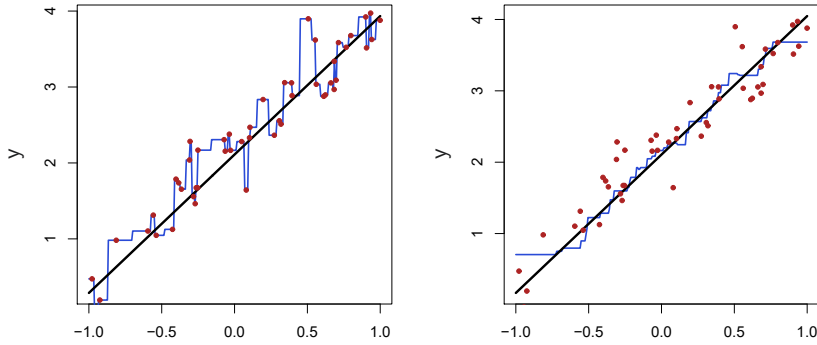
HÌNH 3.2. Đồ thị \hat{f}(X) bằng KNN regression trên dataset một chiều có 50 observation. Quan hệ thực là đường đen liền. Trái: Đường xanh với K = 1 nội suy training data. Phải: Đường xanh với K = 9 cho fit mượt hơn.
