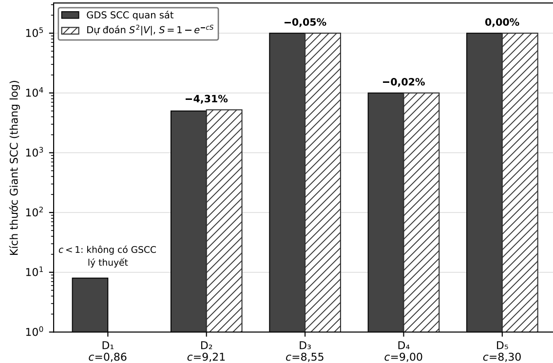
(a) Giant SCC từ benchmark và dự đoán lý thuyết
