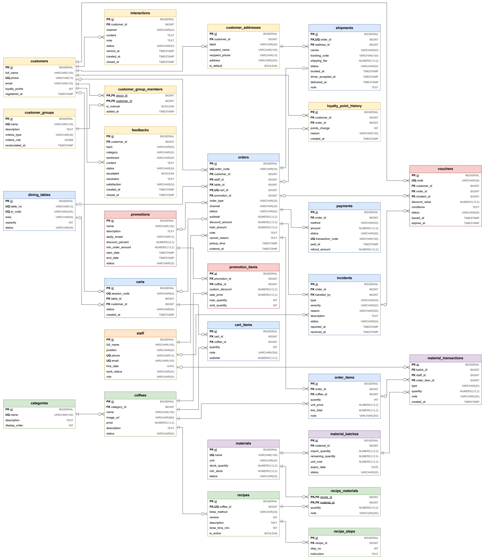
Database diagram (mức vật lý) – PostgreSQL – Website bán cà phê Coffeeholic
