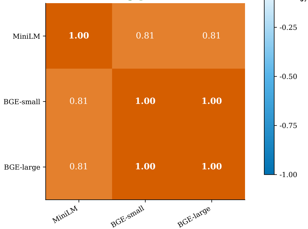
(d) \bar{S}_{div} (Vendi diversity) W = 0.915 (Strong, p = 0.00752)
