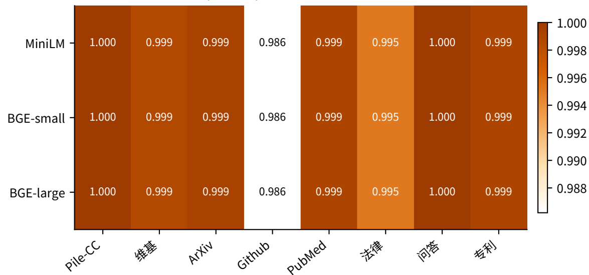
(b) \bar{s}_{num} (有效量) Kendall W = 1.000 (强一致)
