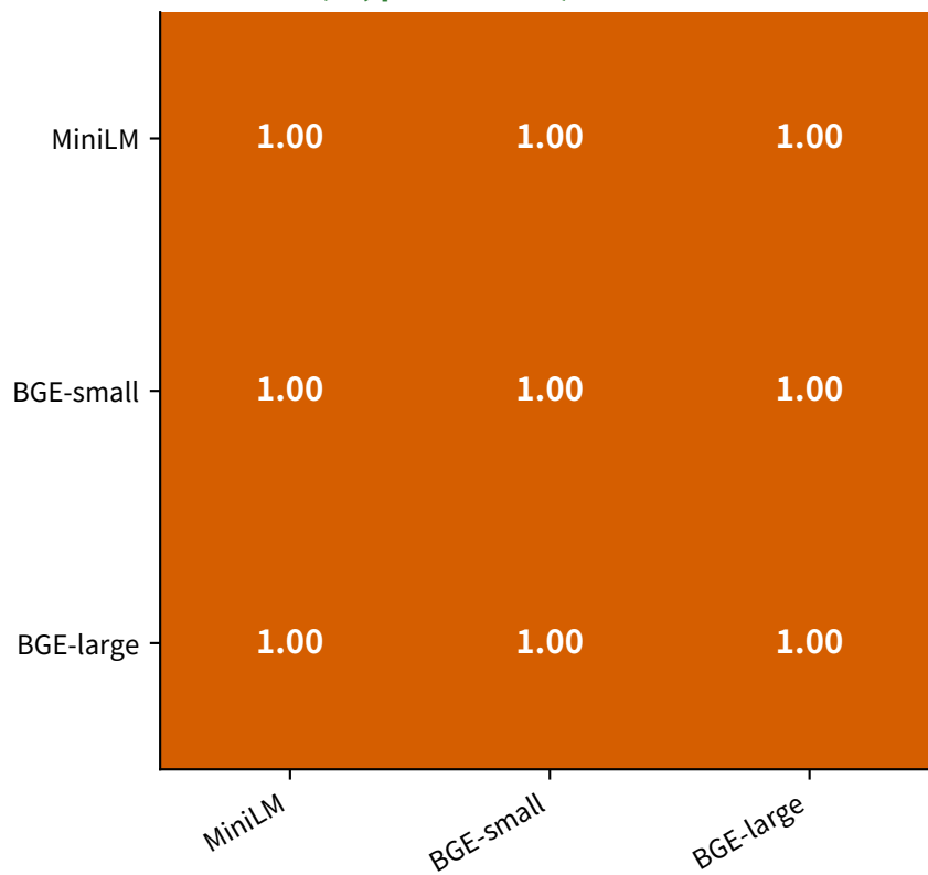
(d) \bar{s}_{div} (Vendi 多样性) W = 0.915 (强, p = 0.00752)
