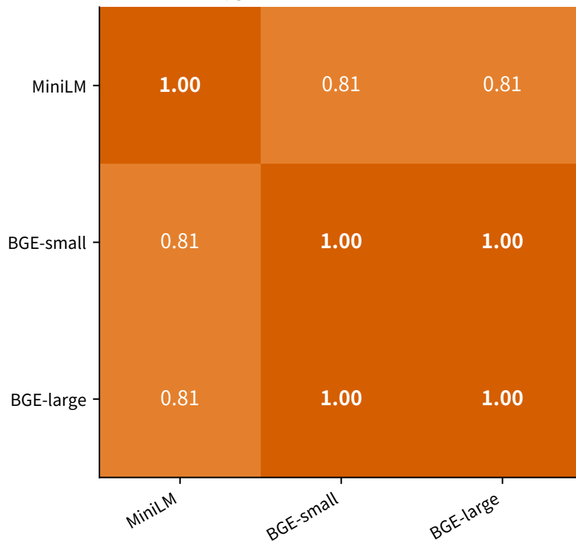
(d) \bar{s}_{div} (Vendi 多样性) W = 0.915 (强, p = 0.00752)
