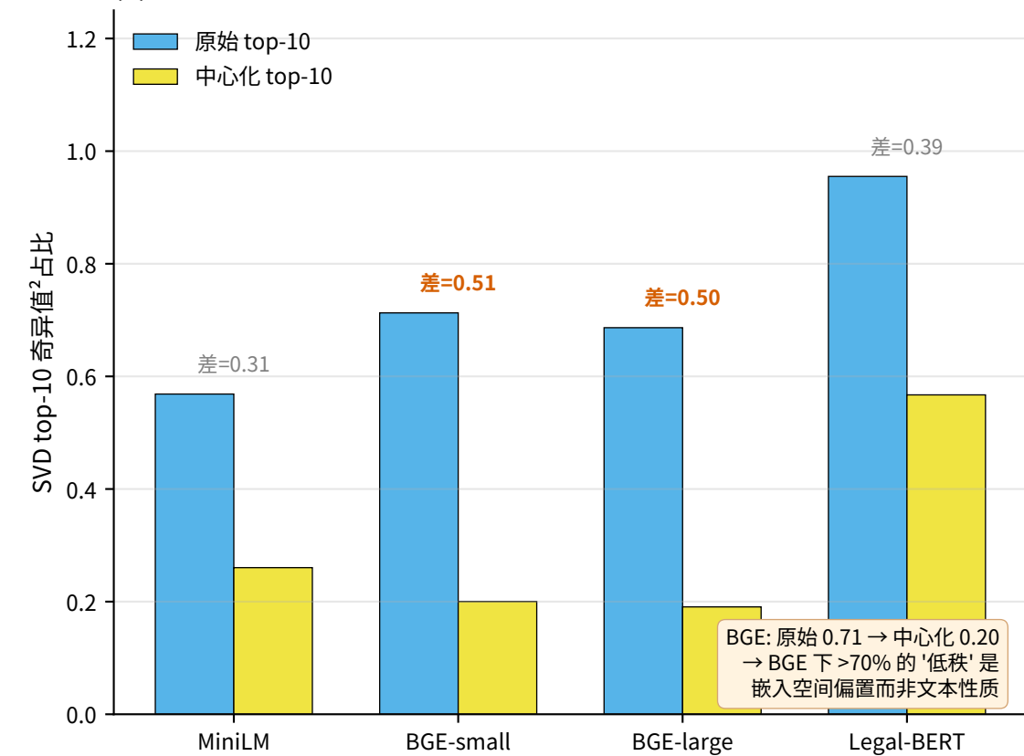
(c) BGE 全局偏置虚影 · 差 \geq 0.50
