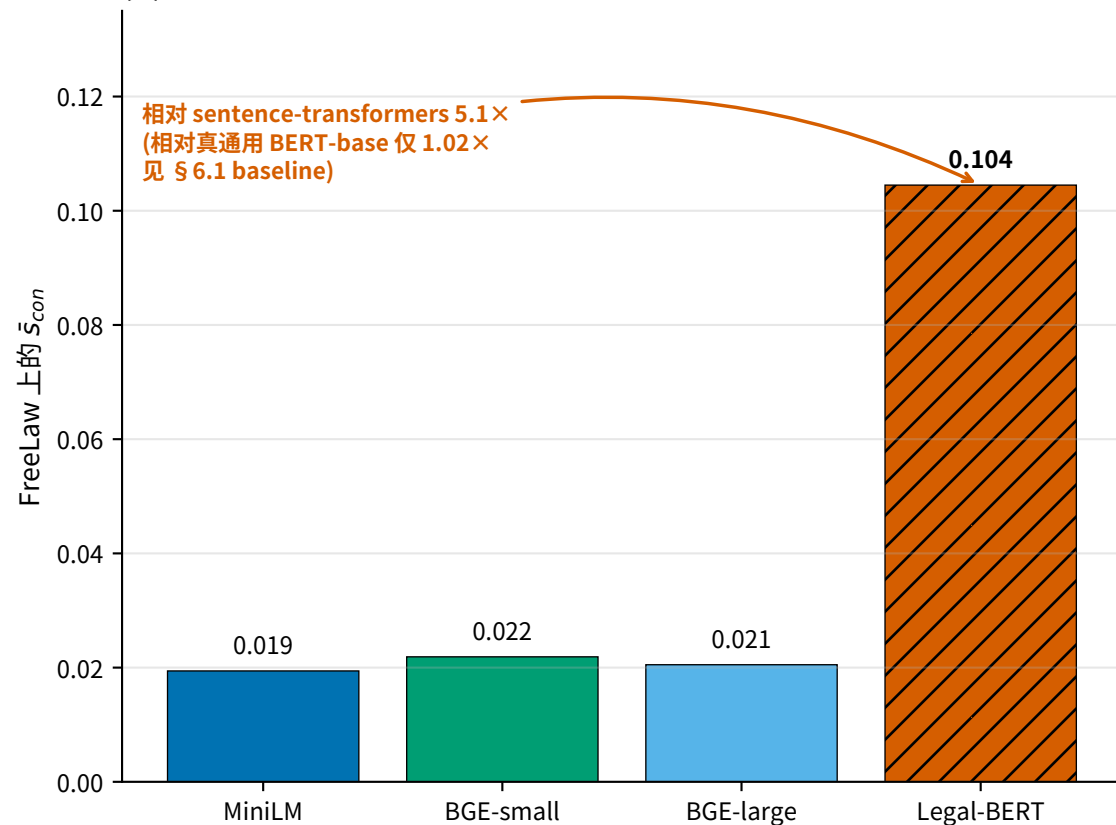
(b) 子类识别 · 法律专模 \neq 通用模型
