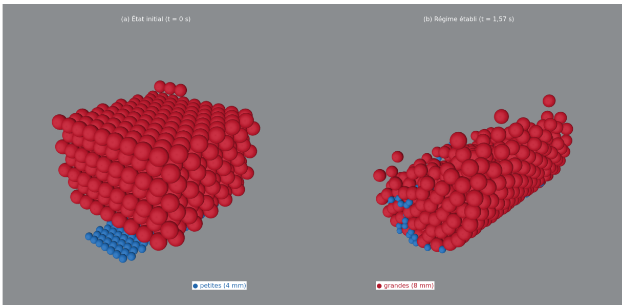
FIGURE 2 – Post-traitement 3D du matériau de référence : les 1030 particules aux diamètres réels (petites 4 mm en bleu, grandes 8 mm en rouge), (a) à l'état initial où les espèces sont séparées et (b) après un tour de tambour, lit en écoulement.
