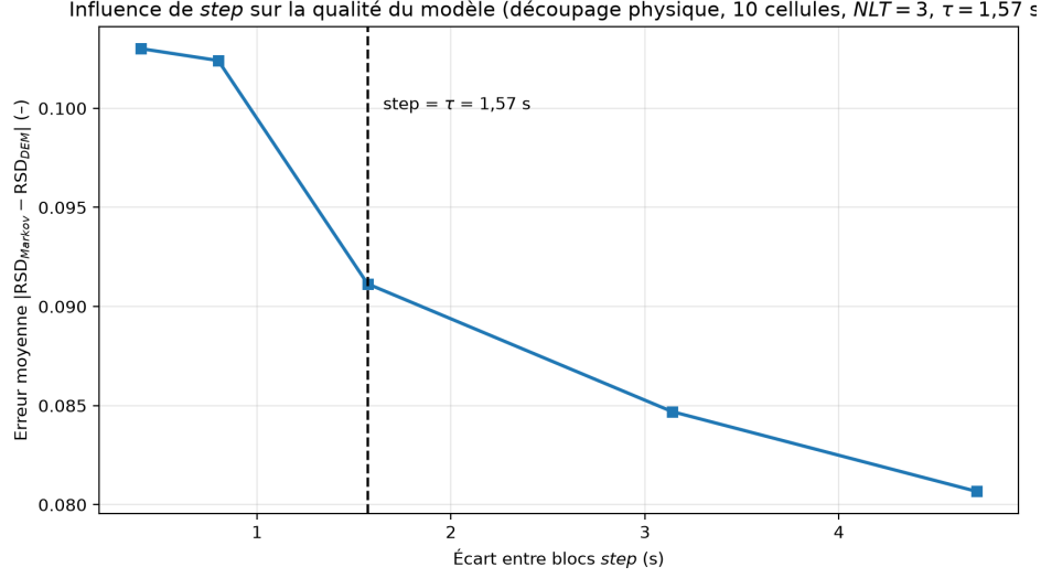
FIGURE 39 – Étude de sensibilité à l'écart entre blocs step , calculée sur les données DEM (découpage physique, 10 cellules, NLT = 3 , \tau = 1,57 s) : erreur moyenne |RSD_{Markov} - RSD_{DEM}| sur la fenêtre de prédiction. La ligne pointillée marque la valeur retenue step = \tau = 1,57 s.
