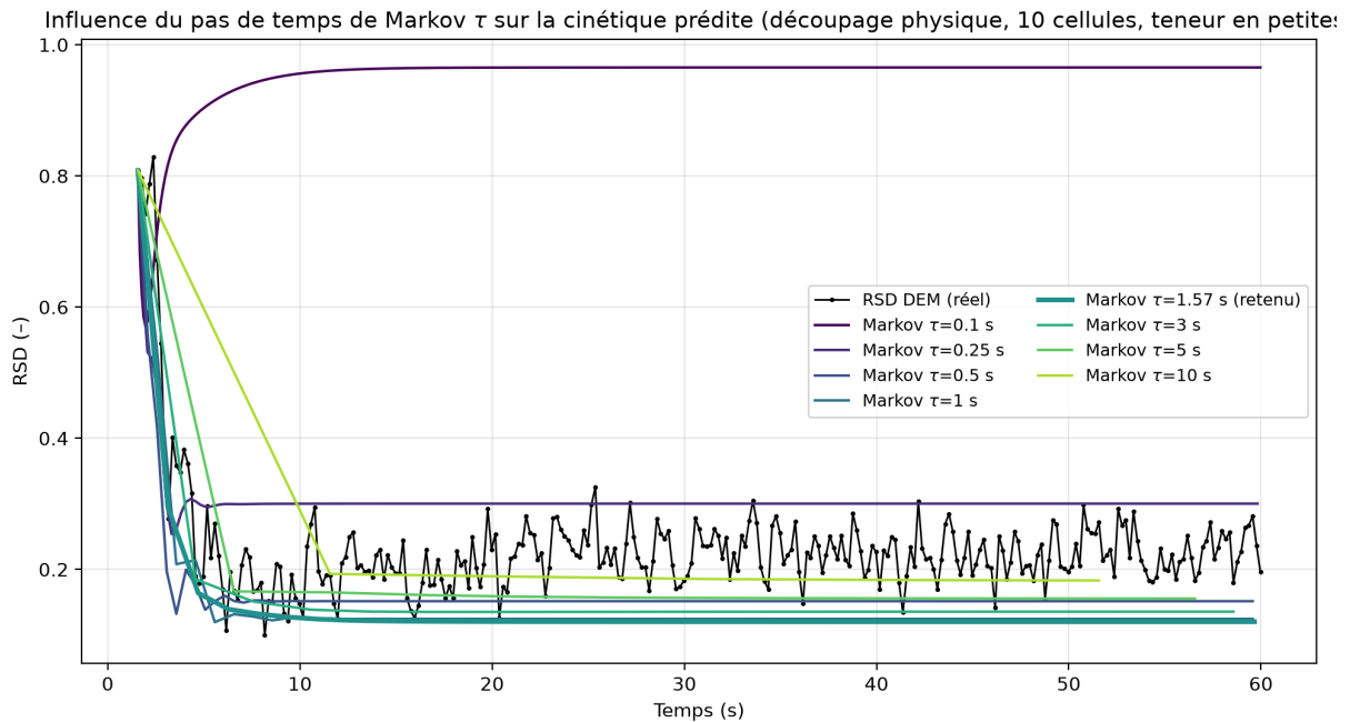
FIGURE 32 – Influence du pas de temps de Markov \tau sur la cinétique de mélange prédite, calculée sur les données DEM (découpage physique, 10 cellules) : RSD DEM de la teneur en petites particules (noir) et prédictions markoviennes homogènes pour \tau de 0,1 s à 10 s. La courbe épaisse correspond à la valeur retenue \tau = 1,57 s.
