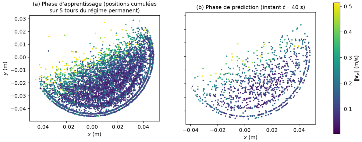
FIGURE 12 – Espace des caractéristiques du découpage physique : positions des 1030 particules colorées par la norme de leur vitesse, (a) cumulées sur la fenêtre d'apprentissage (cinq tours du régime permanent) et (b) à un instant de la phase de prédiction. La zone active de surface (vitesses élevées, teintes claires) se distingue nettement de la zone passive du cœur du lit (vitesses faibles, teintes sombres) : c'est ce contraste que la quatrième caractéristique \|\mathbf{v}_p\| permet de séparer.
