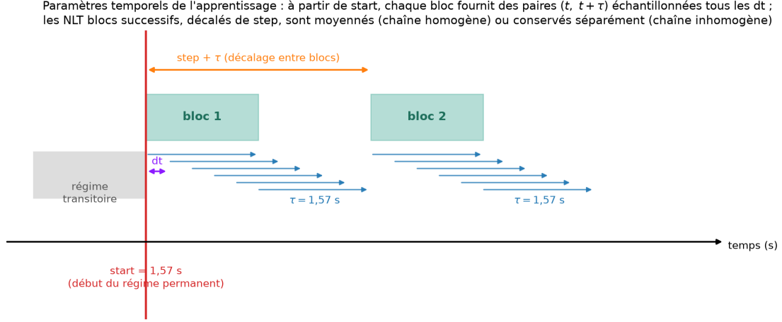
FIGURE 6 – Chronologie des paramètres temporels de l'apprentissage : à partir de start , chaque bloc fournit des paires (t, t + \tau) échantillonnées tous les dt ; les NLT blocs successifs, décalés de step , sont moyennés (chaîne homogène) ou conservés séparément (chaîne inhomogène).
