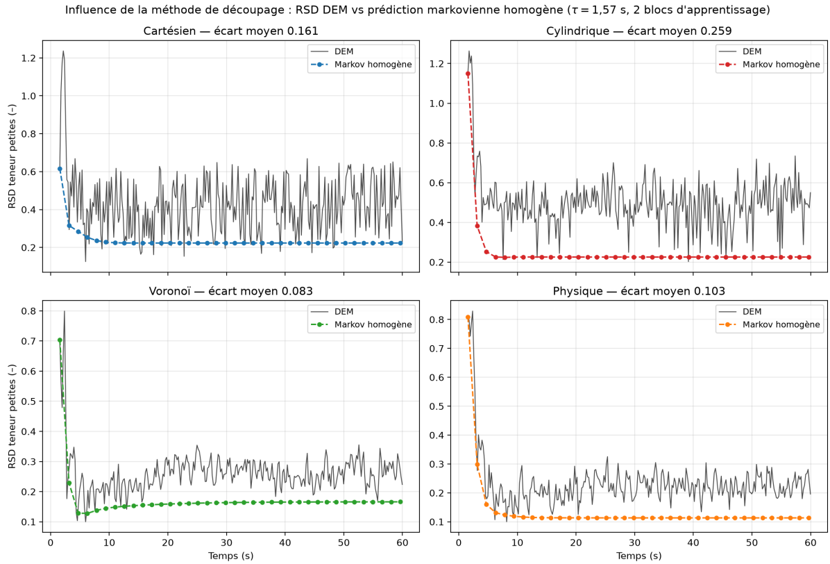
FIGURE 28 – Influence de la méthode de découpage sur la prédiction (données DEM réelles) : RSD DEM vs prédiction markovienne homogène pour les quatre méthodes, à nombre de cellules identique (10 cellules) et à paramètres identiques ( \tau = 1,57 s, deux blocs d'apprentissage). L'écart moyen est indiqué dans le titre de chaque cadran.
