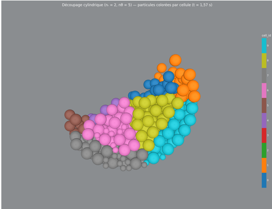
FIGURE 17 – Post-traitement 3D du découpage cylindrique ( n_r = 2, n_\theta = 5 , 10 cellules) : particules aux diamètres réels colorées par le label cell\_id de leur cellule, à t = 1,57 s.
