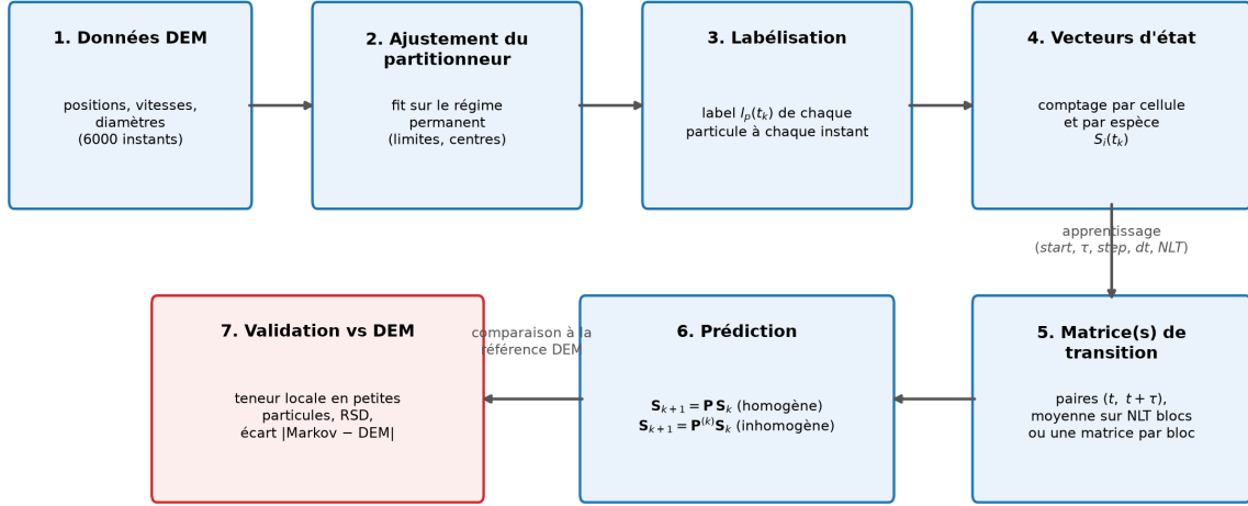
FIGURE 5 – Algorithme de construction et d’exploitation du modèle de Markov : les données DEM servent d’abord à ajuster le partitionneur sur le régime permanent, puis à labelliser chaque particule à chaque instant; les vecteurs d’état de comptage qui en découlent alimentent l’apprentissage de la ou des matrices de transition, la prédiction, et enfin la validation par confrontation à la référence DEM.
