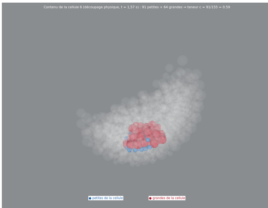
FIGURE 26 – Contenu d’une cellule du découpage physique (cellule la plus peuplée, t = 1,57 s) : les particules de la cellule sont mises en évidence (petites en bleu, grandes en rouge), le reste du lit est estompé. Le dénombrement par espèce donne directement la teneur locale de la cellule.
