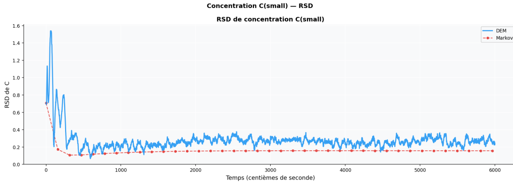
FIGURE 24 – RSD de la concentration en petites particules : comparaison DEM / prédiction markovienne (découpage de Voronoï).
