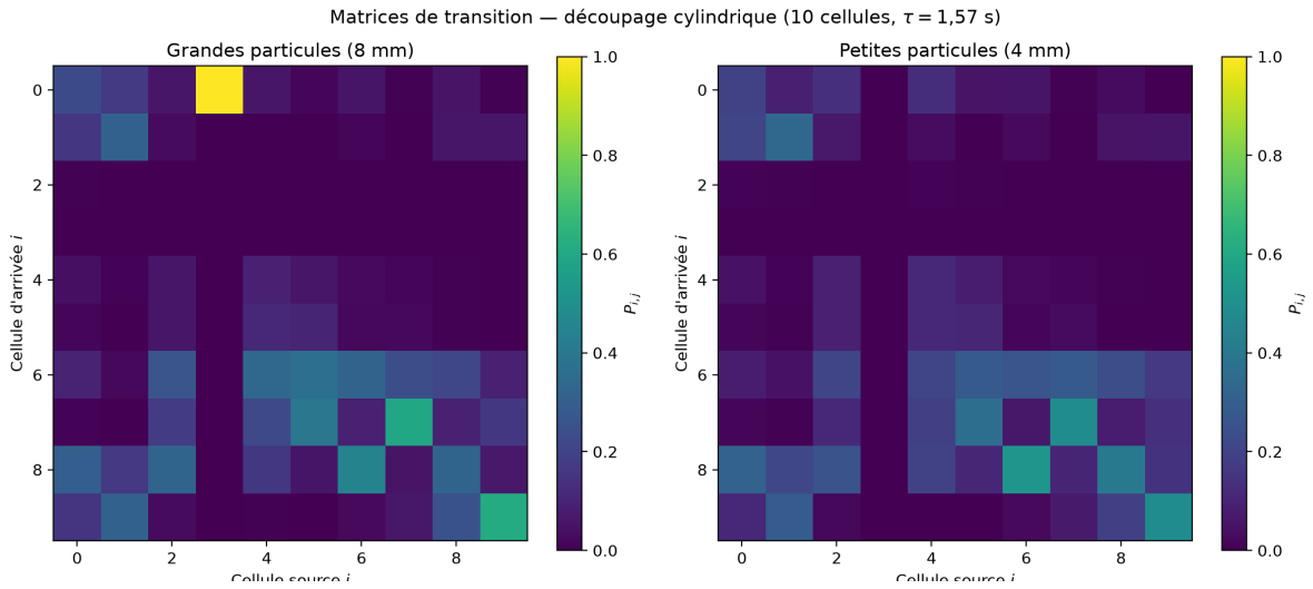
FIGURE 18 – Matrices de transition construites à partir des données DEM pour le découpage cylindrique (10 cellules, n_r = 2 , n_\theta = 5 , mode à aire constante, \tau = 1,57 s), séparément pour chaque espèce. La structure en blocs suit la numérotation radiale \rightarrow angulaire ; la condition de stochasticité en colonne est vérifiée sur toutes les colonnes.
