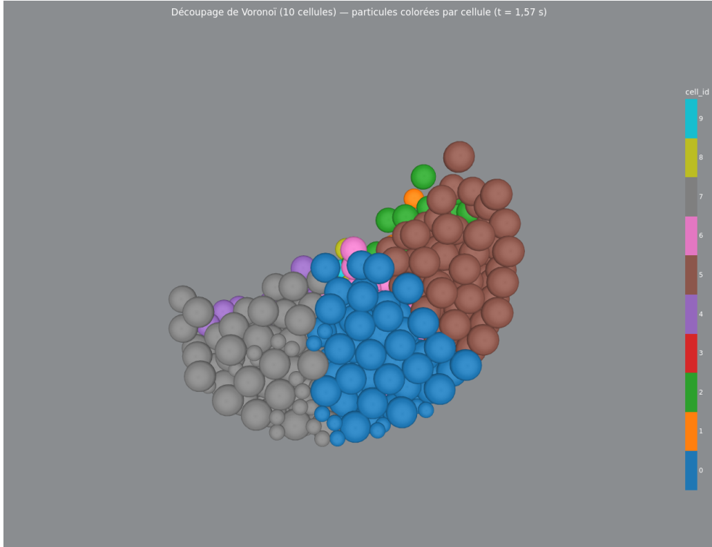
FIGURE 20 – Post-traitement 3D du découpage de Voronoï (10 cellules) : particules aux diamètres réels colorées par le label cell\_id de leur cellule, à t = 1,57 s.
