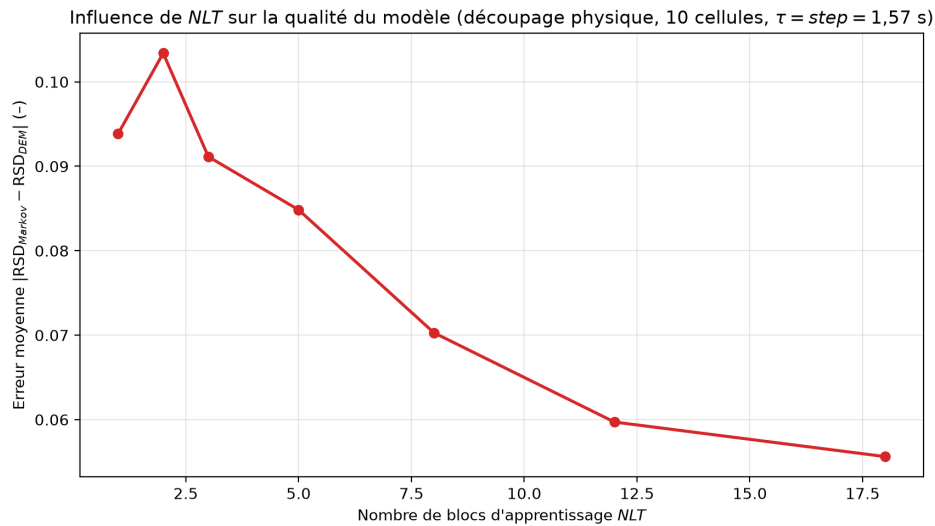
FIGURE 34 – Étude de sensibilité au nombre de blocs d'apprentissage NLT , calculée sur les données DEM (découpage physique, 10 cellules, \tau = step = 1,57 s) : erreur moyenne |RSD_{Markov} - RSD_{DEM}| sur la fenêtre de prédiction.
