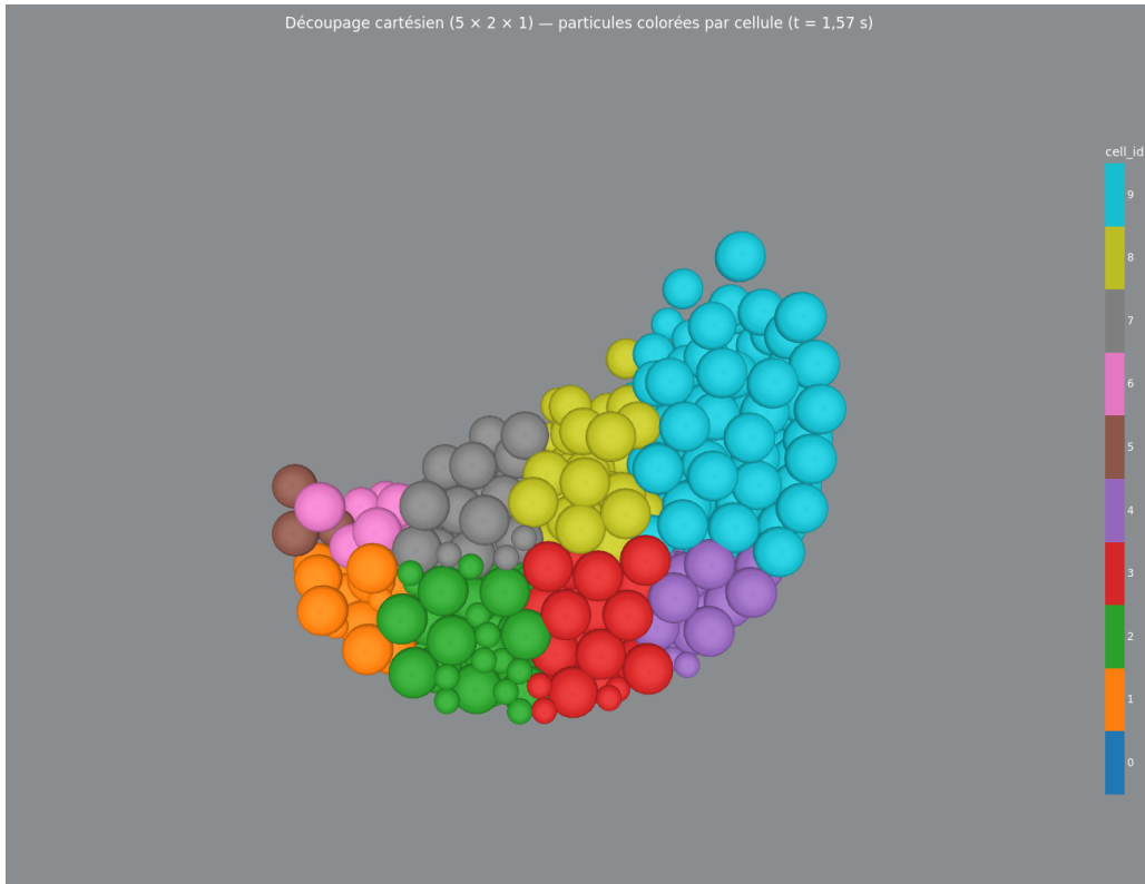
FIGURE 14 – Post-traitement 3D du découpage cartésien ( 5 \times 2 \times 1 , 10 cellules) : particules aux diamètres réels colorées par le label cell_id de leur cellule, à t = 1,57 s.
