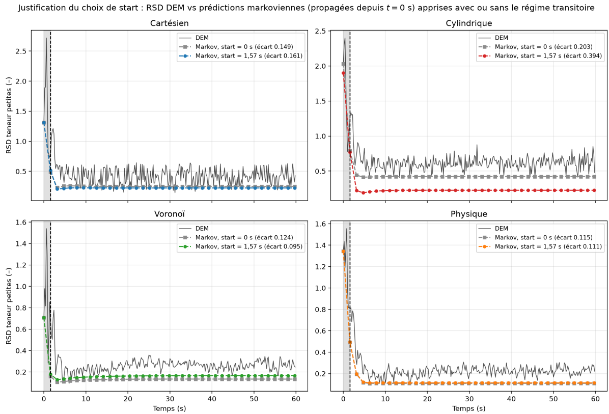
FIGURE 37 – Justification du choix de start : RSD DEM de la teneur en petites particules et prédictions markoviennes homogènes propagées depuis t = 0 s, dont la matrice est apprise soit en incluant le régime transitoire ( start = 0 s, gris), soit sur le régime permanent ( start = 1,57 s, couleur), pour les quatre méthodes de découpage. La zone grisée matérialise le régime transitoire; l'écart moyen |RSD_{Markov} - RSD_{DEM}| est indiqué dans chaque légende.
