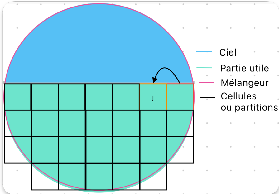
FIGURE 7 – Construction de la matrice de transition à partir des déplacements inter-cellules observés dans le mélangeur discrétisé.
