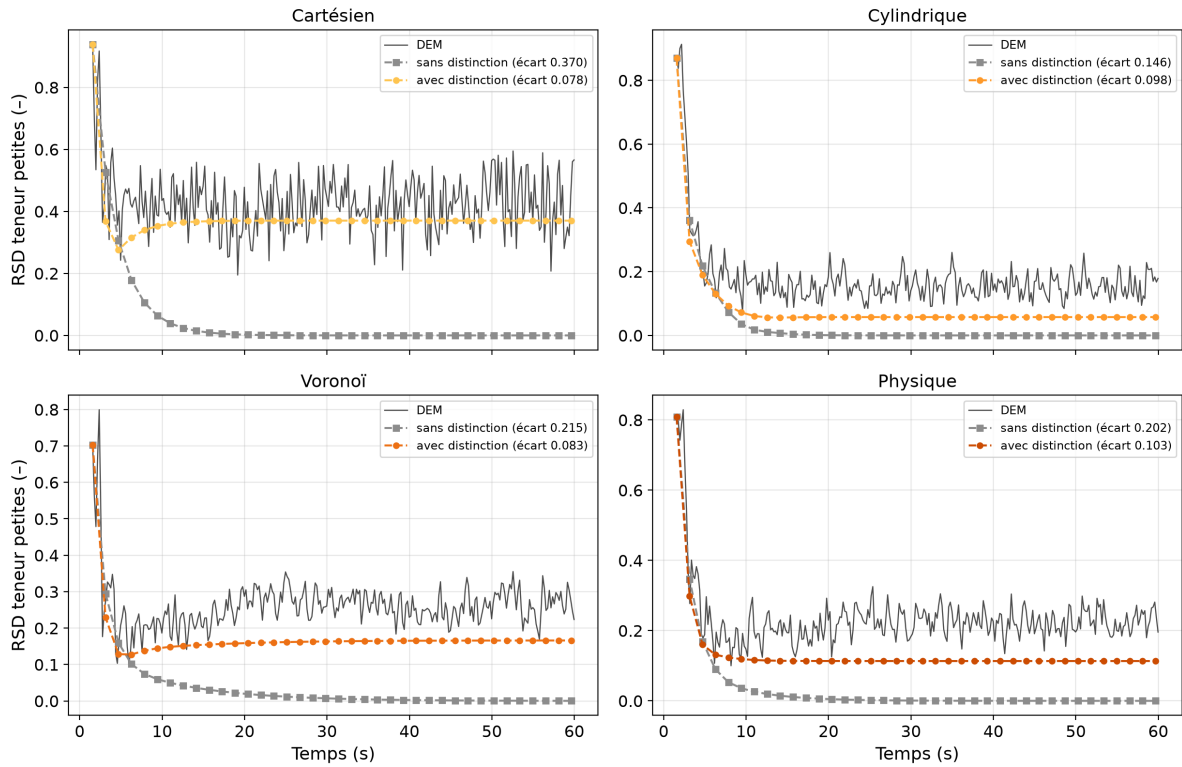
Matrice unique (sans distinction d'espèce) vs matrices par espèce ( \tau = 1,57 s, 2 blocs)
