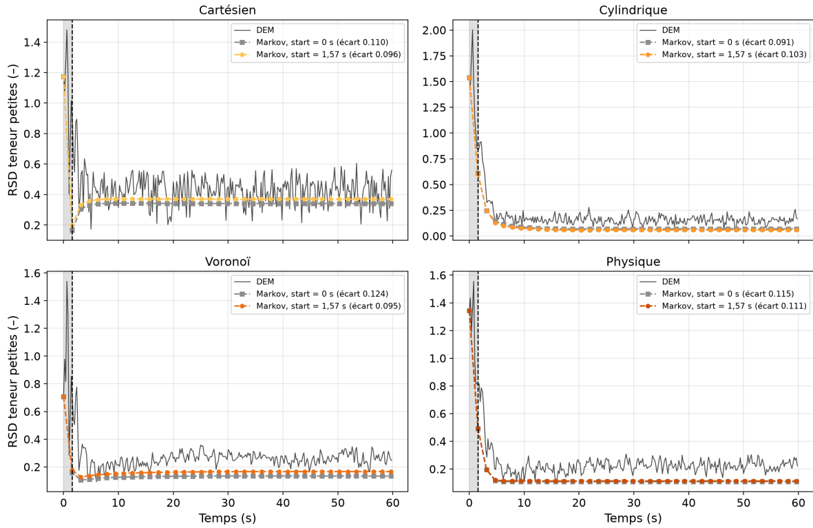
FIGURE 34 – Justification du choix de start : RSD DEM de la teneur en petites particules et prédictions markoviennes homogènes propagées depuis t = 0 s, dont la matrice est apprise soit en incluant le régime transitoire ( start = 0 s, gris), soit sur le régime permanent ( start = 1,57 s, couleur), pour les quatre méthodes de découpage (configuration : nlt = 2 , step = \tau = 1,57 s, dt = 8 pas). La zone grisée matérialise le régime transitoire; l'écart moyen |RSD_{Markov} - RSD_{DEM}| est indiqué dans chaque légende.
