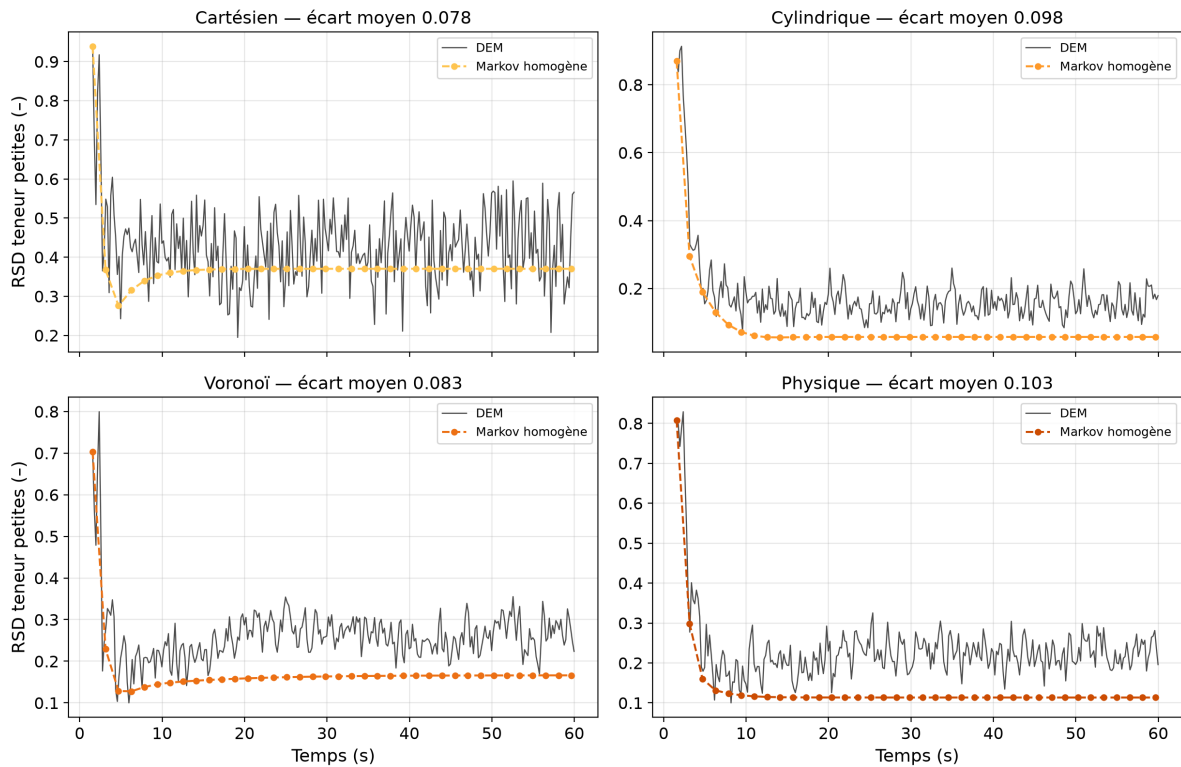
FIGURE 26 – Influence de la méthode de découpage sur la prédiction : RSD DEM vs prédiction markovienne homogène pour les quatre méthodes, à nombre de cellules identique (10 cellules) et à configuration identique ( nlt = 2 , start = 1,57 s, step = \tau = 1,57 s, dt = 8 pas). L'écart moyen est indiqué dans le titre de chaque cadran.
