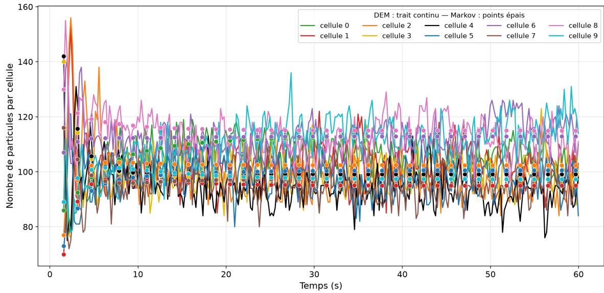
FIGURE 18 – Nombre de particules par cellule (toutes espèces) : référence DEM (trait continu) et prédiction markovienne homogène (marqueurs épais) superposées, une couleur par cellule — découpage de Voronoï, 10 cellules, configuration nlt = 2 , start = 1,57\text{ s} , step = \tau = 1,57\text{ s} , dt = 8\text{ pas} .
