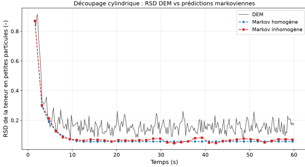
FIGURE 15 – Découpage cylindrique : RSD de la teneur en petites particules, DEM (trait continu) vs prédictions markoviennes homogène ( nlt = 2 ) et inhomogène (une matrice par bloc), configuration start = 1,57 s, step = \tau = 1,57 s, dt = 8 pas.
