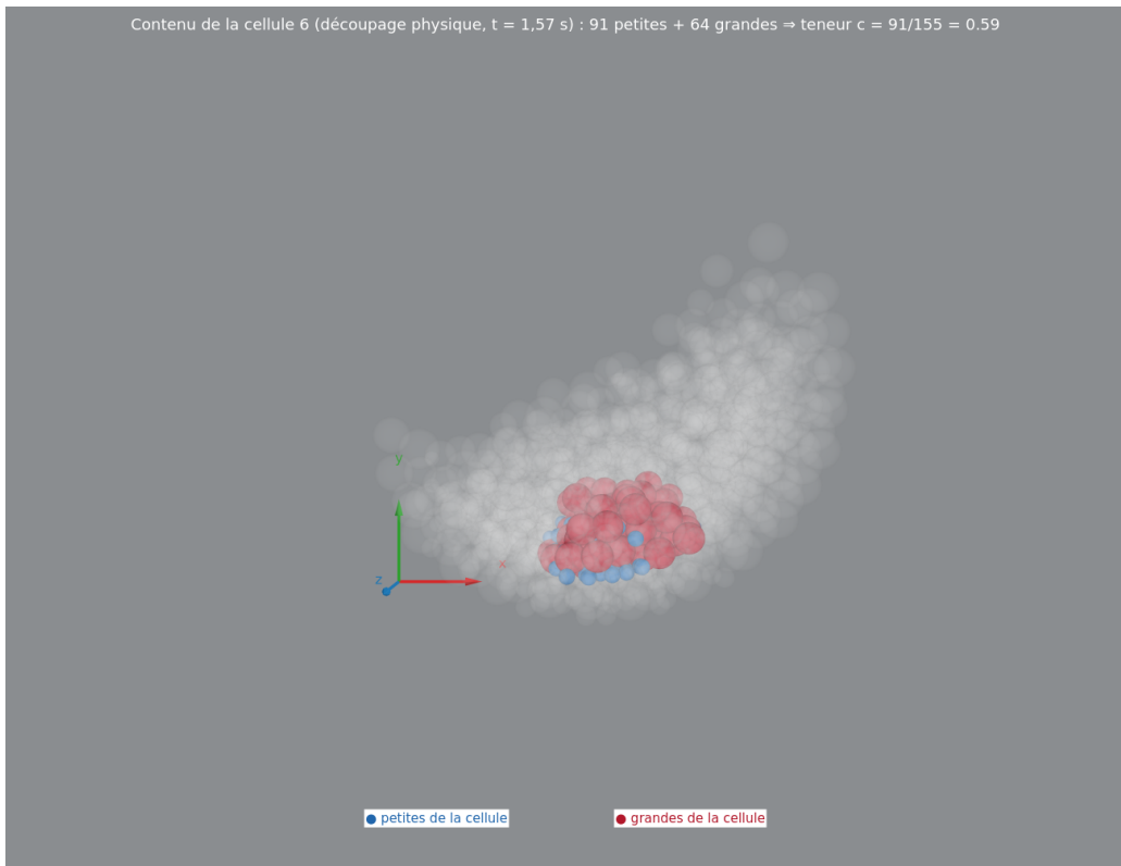
FIGURE 24 – Contenu d'une cellule du découpage physique (cellule la plus peuplée, t = 1,57 s) : les particules de la cellule sont mises en évidence (petites en bleu, grandes en rouge), le reste du lit est estompé. Le dénombrement par espèce donne directement la teneur locale de la cellule.
