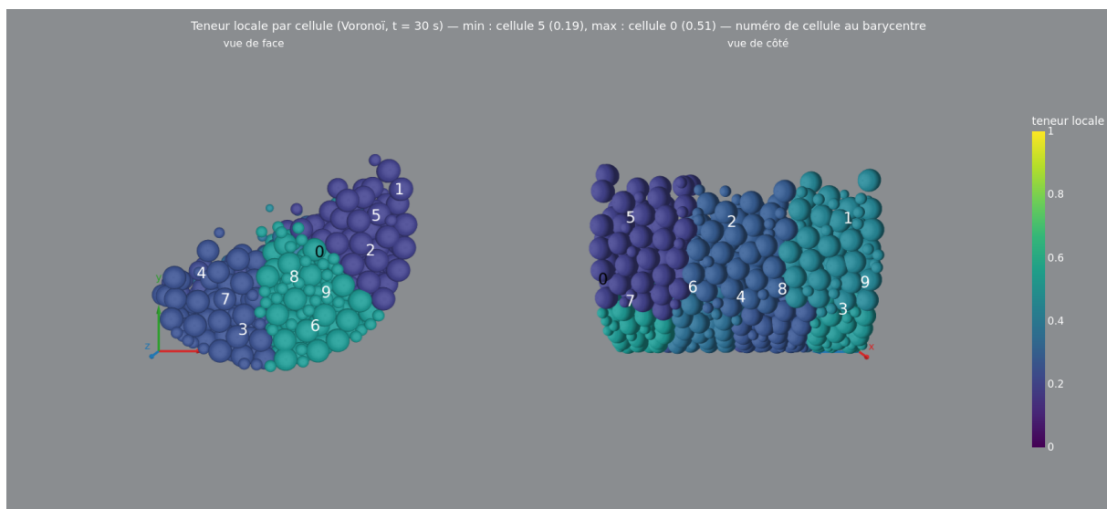
FIGURE 21 – Même représentation à t = 30 s (numéros de cellule aux barycentres) : la gamme de teneurs s'est resserrée mais les cellules du cœur et de la paroi restent enrichies en petites particules, et la surface libre appauvrie — signature spatiale persistante de la ségrégation.
