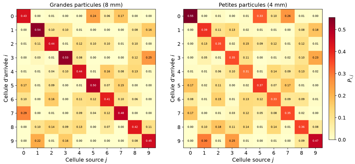
FIGURE 17 – Matrices de transition du découpage de Voronoï (10 cellules, configuration : nlt = 2 , start = 1,57 s , step = \tau = 1,57 s , dt = 8 pas), séparément pour chaque espèce; probabilités arrondies au centième, barre de couleur commune aux deux espèces, chaque colonne somme à un.
