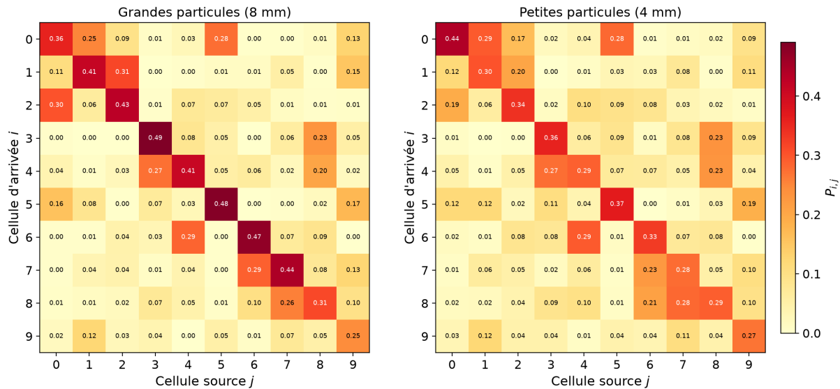
FIGURE 25 – Matrices de transition du découpage physique (10 cellules, configuration : nlt = 2 , start = 1,57\text{ s} , step = \tau = 1,57\text{ s} , dt = 8\text{ pas} ), séparément pour chaque espèce; probabilités arrondies au centième, barre de couleur commune aux deux espèces, chaque colonne somme à un.
