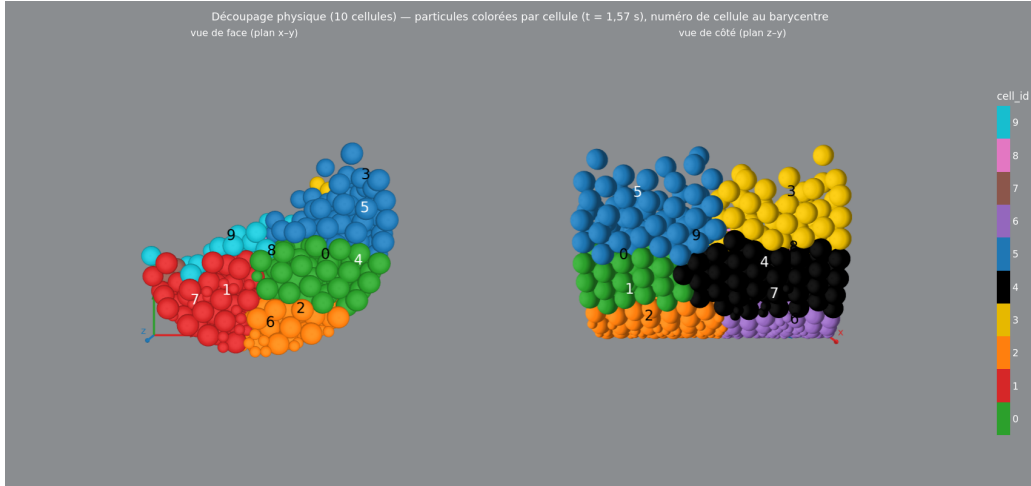
FIGURE 23 – Découpage physique (10 cellules) : particules aux diamètres réels colorées par le label cell\_id (numéro de cellule au barycentre), vue de face et vue de côté, à t = 1,57 s. Le vecteur de caractéristiques (positions + vitesse relative) produit des cellules stratifiées entre surface libre et cœur du lit, partagées aussi selon l'axe z .
