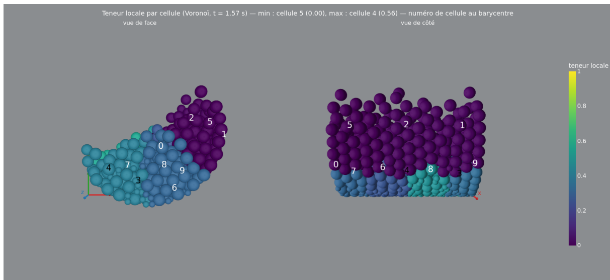
FIGURE 20 – Mélangeur discrétisé (Voronoi, labels et teneurs calculés sur la configuration de référence nlt = 2 , start = 1,57 s, step = \tau = 1,57 s, dt = 8 pas) coloré par la teneur locale de chaque cellule à t = 1,57 s, vues de face et de côté; le numéro de chaque cellule est inscrit à son barycentre. Les cellules héritées de la couche initiale de petites particules contrastent avec les cellules du haut du lit, quasi vides de petites particules.
