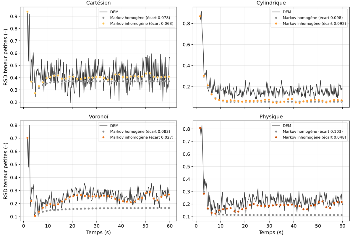
FIGURE 28 – RSD de la teneur en petites particules : référence DEM (trait continu) et prédictions markoviennes homogène (gris) et inhomogène (couleur), en marqueurs épais, superposées sur une même figure pour chacune des quatre méthodes de découpage (10 cellules chacune, start = 1,57 s, step = \tau = 1,57 s, dt = 8 pas; chaîne inhomogène : une matrice par tour de tambour). L'écart moyen |RSD_{Markov} - RSD_{DEM}| est indiqué dans chaque légende.
