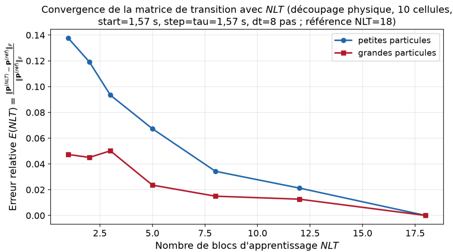
FIGURE 31 – Étude de sensibilité au nombre de blocs d'apprentissage NLT par l'erreur relative sur la matrice de transition (équation (19), grandeur de comparaison de Doucet et al. [5]) : découpage physique, 10 cellules, configuration start = 1,57 s, step = \tau = 1,57 s, dt = 8 pas, référence NLT_{\text{réf}} = 18 .
