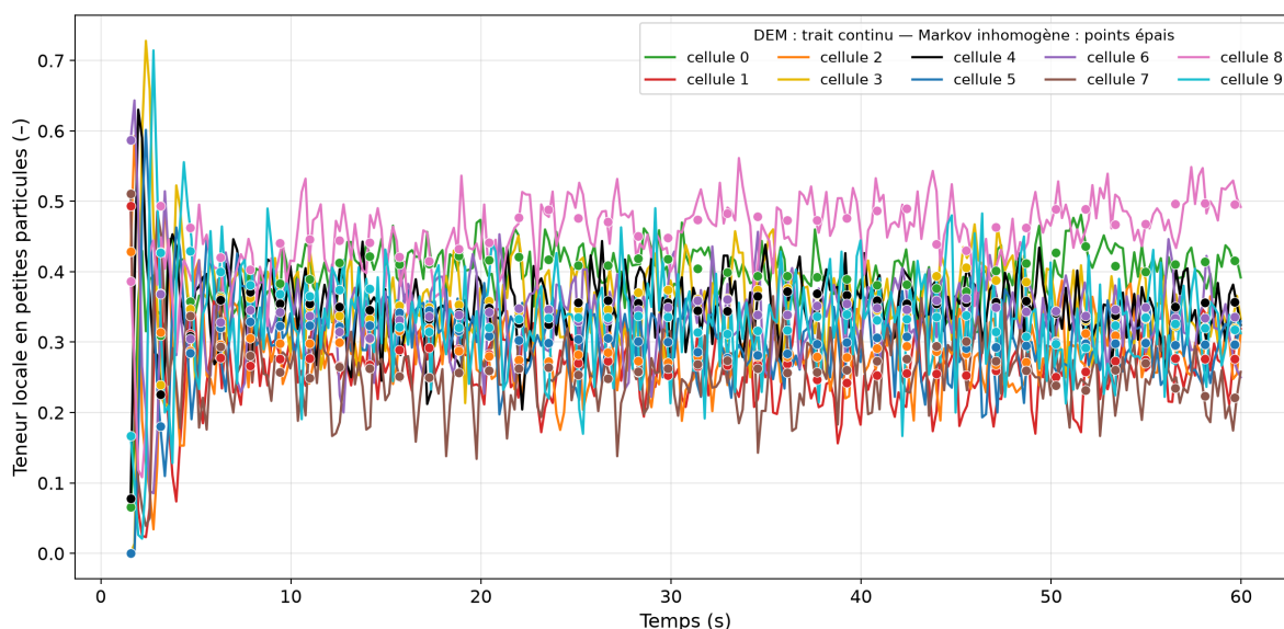
FIGURE 27 – Teneur locale en petites particules par cellule : référence DEM (trait continu) et prédiction de la chaîne inhomogène (marqueurs épais) superposées, une couleur par cellule — découpage physique, 10 cellules, configuration start = 1,57\text{ s} , step = \tau = 1,57\text{ s} , dt = 8\text{ pas} , une matrice par tour de tambour.
