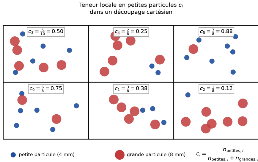
FIGURE 38 – Illustration de la teneur locale en petites particules c_i dans un découpage cartésien : rapport du nombre de petites particules (bleu) au nombre total de particules de la cellule. Les écarts de teneur entre cellules signent la ségrégation.
