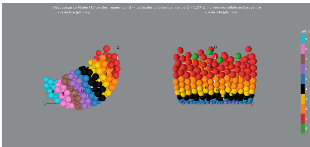
FIGURE II – Découpage cartésien (10 bandes dans le repère du lit) : particules aux diamètres réels colorées par le label cell_id (numéro de cellule au barycentre), vue de face et vue de côté, à t = 1,57 s. Les bandes suivent la direction principale du lit; chacune traverse son épaisseur et couvre toute la longueur axiale.
