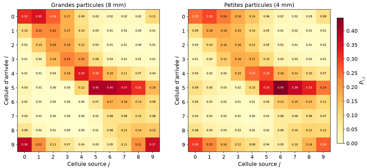
FIGURE 14 – Matrices de transition du découpage cylindrique (10 secteurs angulaires dans le repère du lit; configuration : nlt = 2 , start = 1,57 s, step = \tau = 1,57 s, dt = 8 pas), séparément pour chaque espèce; probabilités arrondies au centième, barre de couleur commune aux deux espèces, chaque colonne somme à un.
