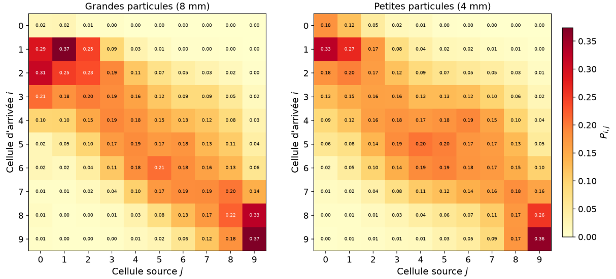
FIGURE 12 – Matrices de transition du découpage cartésien (10 bandes dans le repère du lit; configuration : nlt = 2 , start = 1,57 s, step = \tau = 1,57 s, dt = 8 pas), séparément pour chaque espèce; probabilités arrondies au centième, barre de couleur commune aux deux espèces, chaque colonne somme à un.
