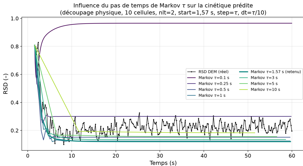
FIGURE 30 – Influence du pas de temps de Markov \tau sur la cinétique de mélange prédite, calculée sur les données de la simulation (découpage physique, 10 cellules; configuration : nlt = 2 , start = 1,57 s, step = \tau , dt = \tau/10 ) : RSD DEM de la teneur en petites particules (noir) et prédictions markoviennes homogènes pour \tau de 0,1 s à 10 s. La courbe épaisse correspond à la valeur retenue \tau = 1,57 s.
