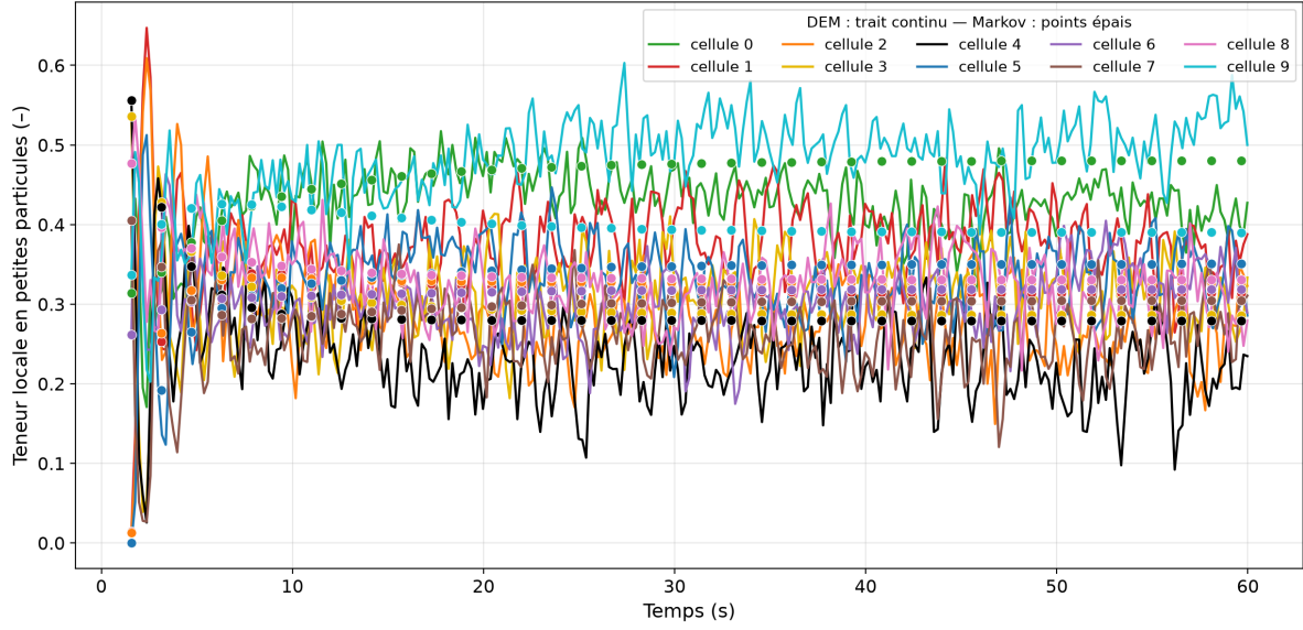
FIGURE 19 – Teneur locale en petites particules par cellule : référence DEM (trait continu) et prédiction markovienne homogène (marqueurs épais) superposées, une couleur par cellule — découpage de Voronoï, 10 cellules, configuration nlt = 2 , start = 1,57 s, step = \tau = 1,57 s, dt = 8 pas.
