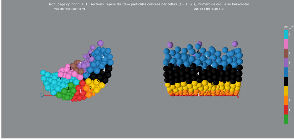
FIGURE 13 – Découpage cylindrique (10 secteurs angulaires dans le repère du lit) : particules aux diamètres réels colorées par le label cell_id (numéro de cellule au barycentre), vue de face et vue de côté, à t = 1,57 s. Les secteurs centrés sur le barycentre du lit se lisent sur la vue de face ; chacun est occupé en permanence.
