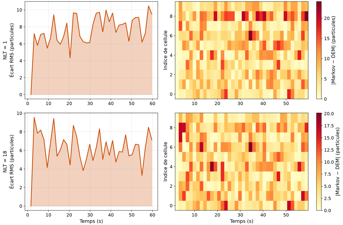
FIGURE 32 – Influence du nombre de blocs d'apprentissage NLT sur la qualité du modèle (découpage physique, 10 cellules, petites particules, configuration start = 1,57 s, step = \tau = 1,57 s, dt = 8 pas) : écart temporel RMS |\text{Markov} - \text{DEM}| (gauche) et carte des écarts absolus par cellule (droite), pour NLT = 1 (haut) et NLT = 18 , seuil de convergence de la matrice (bas).
