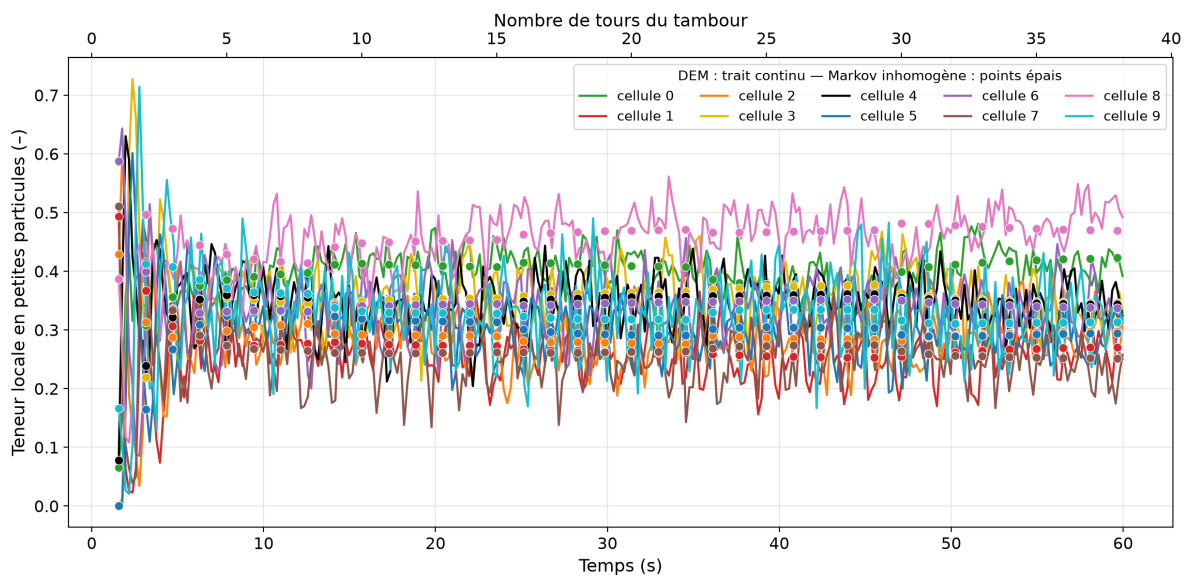
FIGURE 32 – Teneur locale en petites particules par cellule : référence DEM et prédiction de la chaîne inhomogène, découpage physique, 10 cellules ( start = 1,57 s, \tau = 1,57 s, dt = 8 pas; blocs espacés de 7 tours, soit 5 matrices). Légende normale, pointillés réduits.
