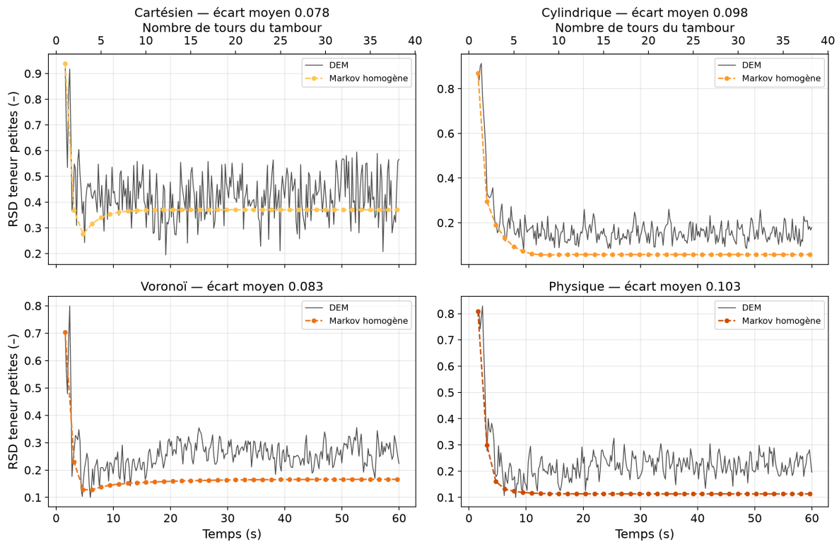
FIGURE 30 – Influence de la méthode de découpage sur la prédiction : RSD DEM vs prédiction markovienne homogène pour les quatre méthodes, à nombre de cellules identique (10 cellules) et à configuration identique ( nlt = 2 , start = 1,57 s, step = \tau = 1,57 s, dt = 8 pas).
