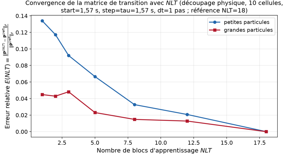
FIGURE 36 – Étude de sensibilité au nombre de blocs d'apprentissage NLT par l'erreur relative sur la matrice de transition (équation (??), grandeur de comparaison de Doucet et al. [5]) : découpage physique, 10 cellules, configuration start = 1,57 s, step = \tau = 1,57 s, dt = 1 pas, référence NLT_{\text{réf}} = 18 .
