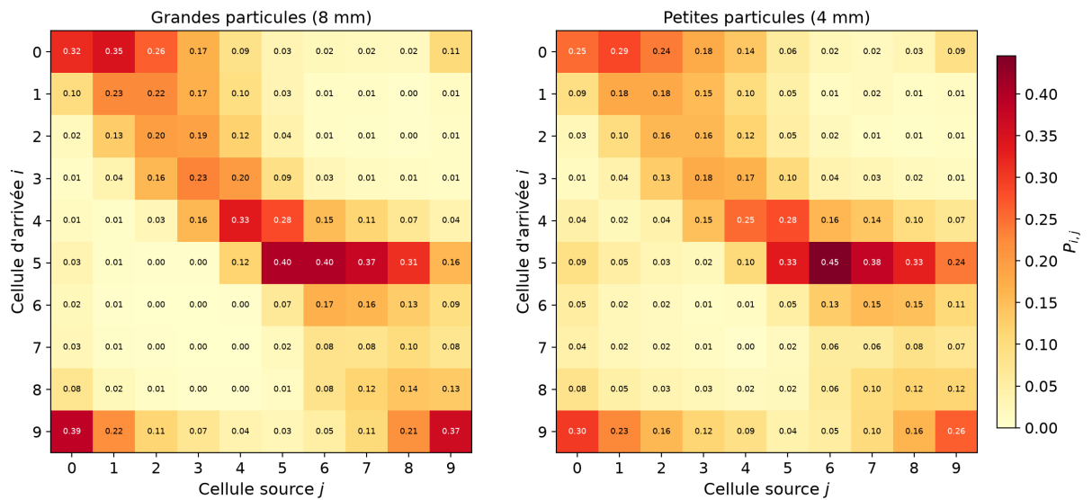
FIGURE 17 – Matrices de transition du découpage cylindrique (10 secteurs angulaires dans le repère du lit; configuration : nlt = 2 , start = 1,57 s, step = \tau = 1,57 s, dt = 8 pas),
