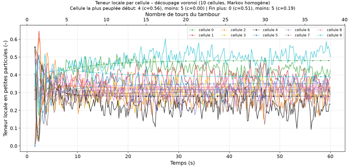
FIGURE 22 – Teneur locale en petites particules par cellule Voronoï au cours du temps, 10 cellules, configuration nlt = 2 , start = 1,57 s, step = \tau = 1,57 s, dt = 8 pas. Légende normale, pointillés Markov de taille réduite. Cellule la plus peuplée début : 4 ( c = 0,56 ), moins : 5 ( c = 0,00 ); fin plus : 0 ( c = 0,51 ), moins : 5 ( c = 0,19 ).
