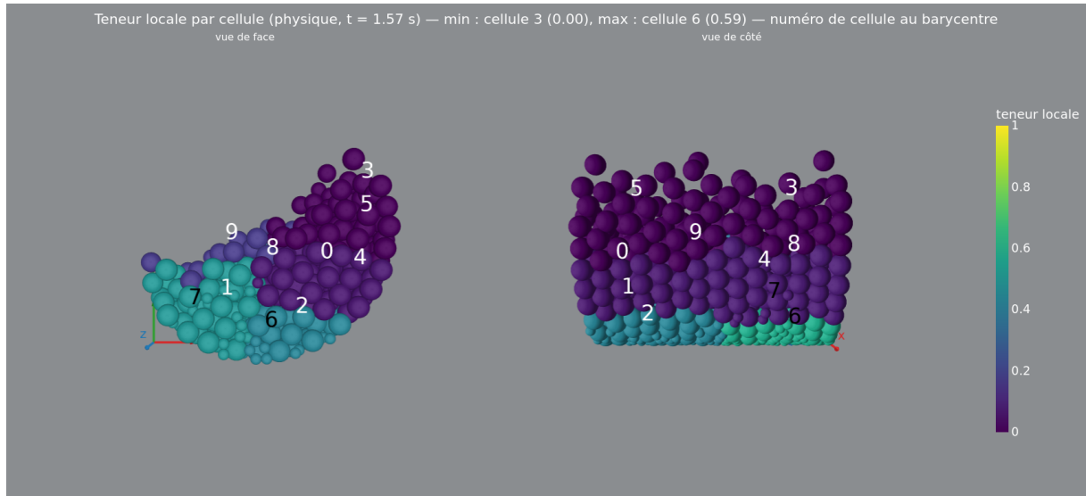
FIGURE 28 – Mélangeur discrétisé par le découpage physique, zoom cadré, coloré par la teneur locale de chaque cellule à t = 1,57 s, vues de face et de côté; numéro de cellule au barycentre (configuration : nlt = 2 , start = 1,57 s, step = \tau = 1,57 s, dt = 8 pas). Cellules les plus peuplées : cœur passif; les moins peuplées : surface active.
