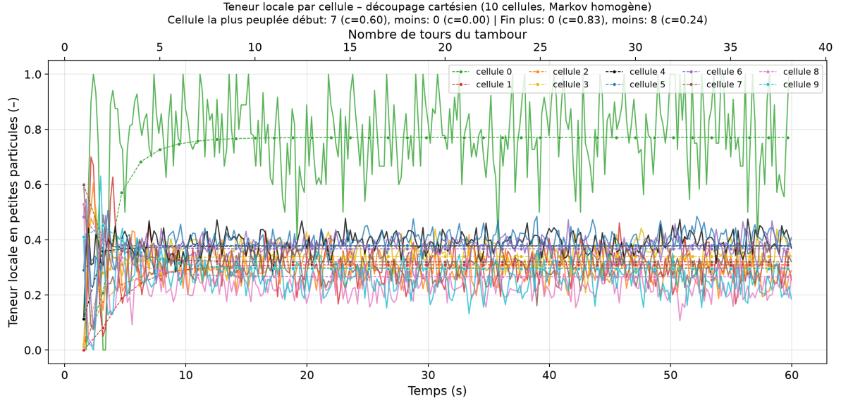
FIGURE 15 – Évolution de la teneur locale en petites particules au cours du temps – découpage cartésien (10 bandes, Markov homogène, n_{lt} = 2 , start = 1,57s , step = \tau = 1,57s , dt = 8 pas). Légende normale, pointillés Markov de taille réduite. Cellule la plus peuplée début : 7, moins : 0 ; fin plus : 0, moins : 8.
