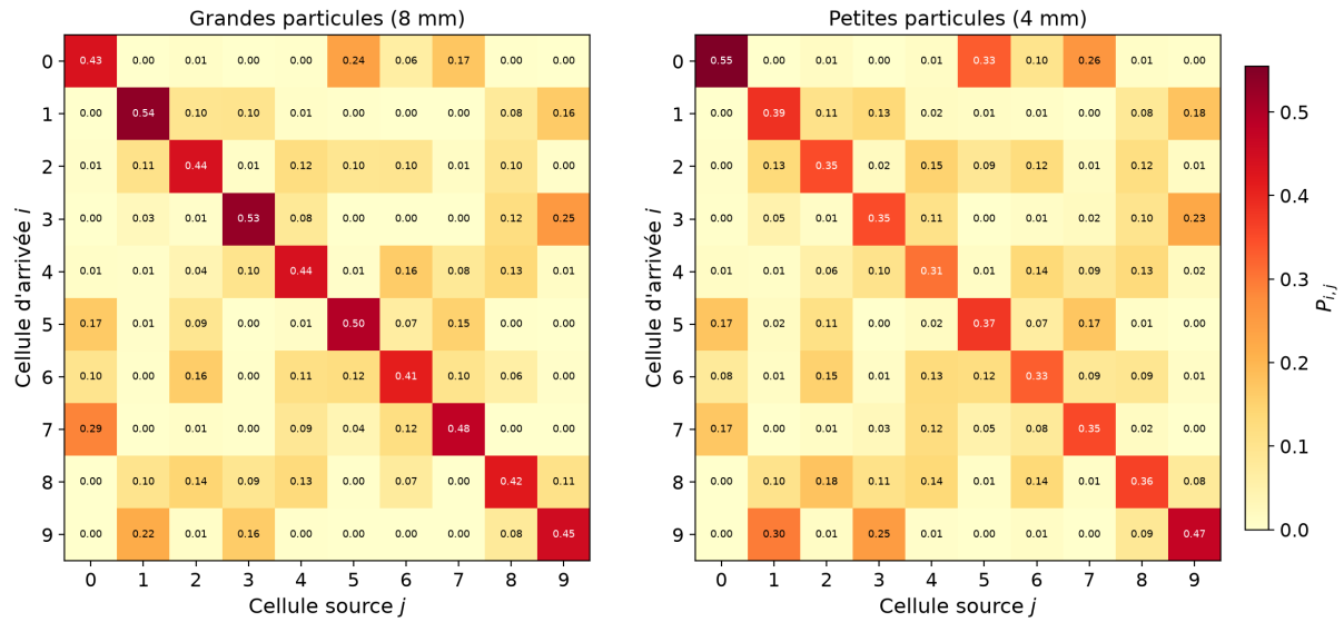
FIGURE 21 – Matrices de transition du découpage de Voronoï (10 cellules, configuration : nlt = 2 , start = 1,57 s , step = \tau = 1,57 s , dt = 8 pas ).
