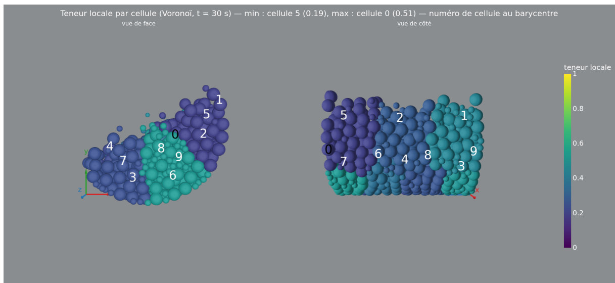
FIGURE 24 – Même représentation à t = 30 s, zoom cadré. Cellules les plus peuplées : 0 et 9 (cœur et paroi); la moins peuplée : 5 (surface libre).
