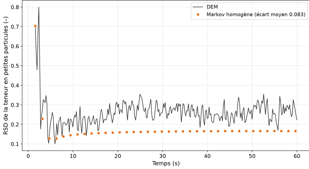
FIGURE 25 – RSD de la concentration en petites particules, découpage de Voronoï, 10 cellules, configuration nlt = 2 , start = 1,57 s, step = \tau = 1,57 s, dt = 8 pas. Légende normale.
