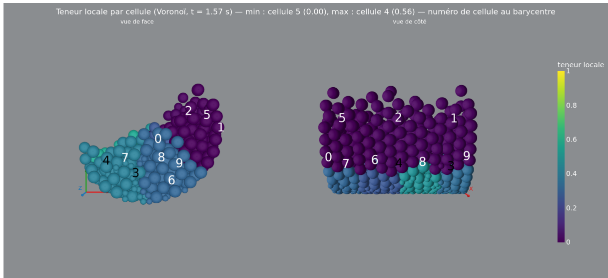
FIGURE 23 – Mélangeur discrétisé en cellules de Voronoï, zoom cadré, sur la configuration de référence nlt = 2 , start = 1,57 s, step = \tau = 1,57 s, dt = 8 pas. Cellule la plus peuplée : 4.
