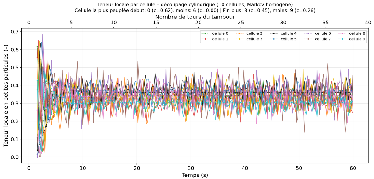
FIGURE 19 – Évolution de la teneur locale en petites particules au cours du temps – découpage cylindrique (10 secteurs, Markov homogène). Légende normale, pointillés réduits. Plus peuplée début : 0, moins : 6 ; fin plus : 3, moins : 9.
