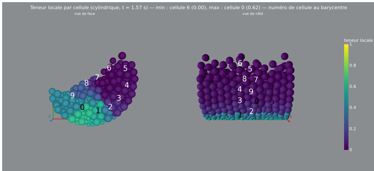
FIGURE 18 – Mélangeur discrétisé en secteurs cylindriques (repère du lit) coloré par la teneur locale de chaque cellule à t = 1,57 s, vues de face et de côté; numéro de cellule au barycentre (configuration : nlt = 2 , start = 1,57 s, step = \tau = 1,57 s, dt = 8 pas).
