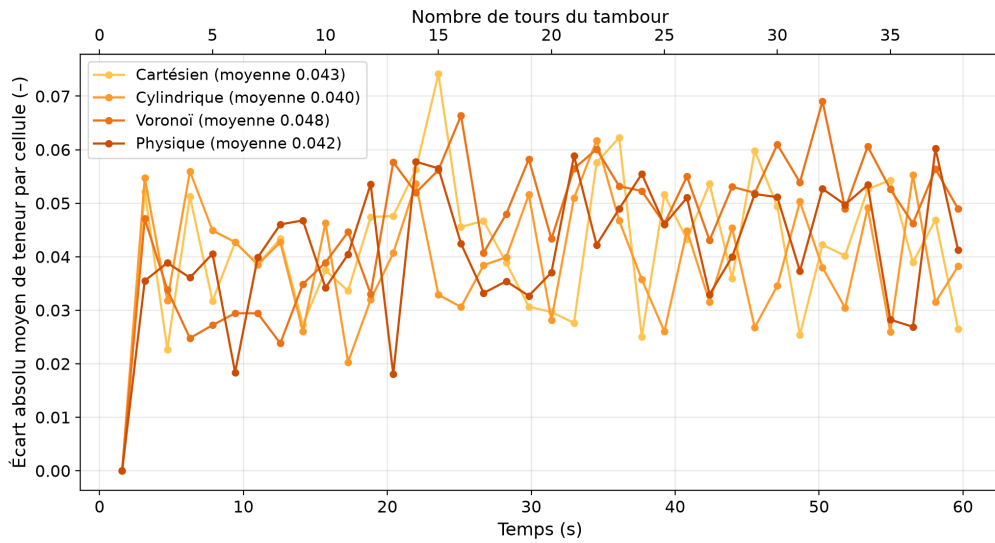
FIGURE 31 – Approche globale sur les courbes de teneur : écart absolu moyen de teneur par cellule entre la prédiction markovienne homogène et la référence DEM, pour les quatre méthodes de découpage à nombre de cellules identique (10 cellules, configuration nlt = 2 , start = 1,57 s, step = \tau = 1,57 s, dt = 8 pas).
