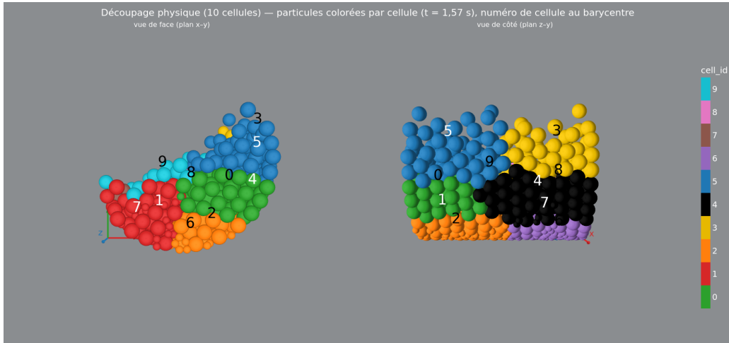
FIGURE 26 – Découpage physique (10 cellules), zoom cadré, à t = 1,57 s. Les cellules suivent les iso-vitesses : cœur lent vs surface rapide.
