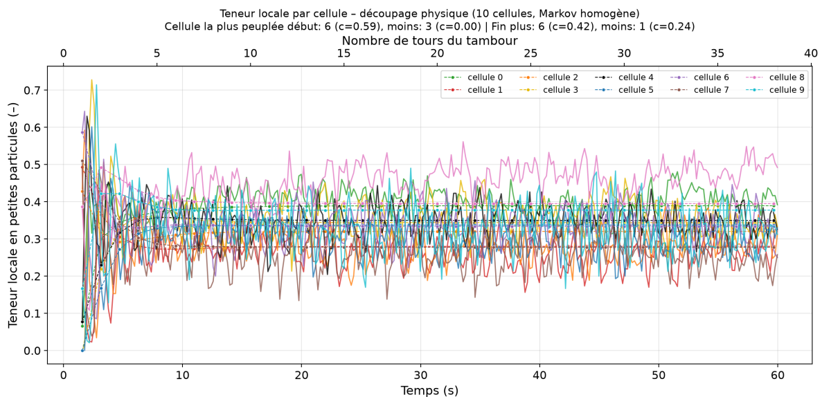
FIGURE 29 – Évolution de la teneur locale en petites particules au cours du temps – découpage physique (10 cellules, Markov homogène). Légende normale, pointillés réduits. Plus peuplée début : 6, moins : 3; fin plus : 6, moins : 1.
