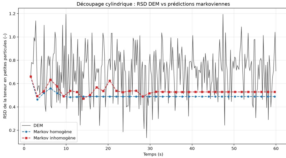
FIGURE 16 – Découpage cylindrique : RSD de la teneur en petites particules, DEM (trait continu) vs prédictions markoviennes homogène et inhomogène ( \tau = 1,57 s, données DEM réelles).
