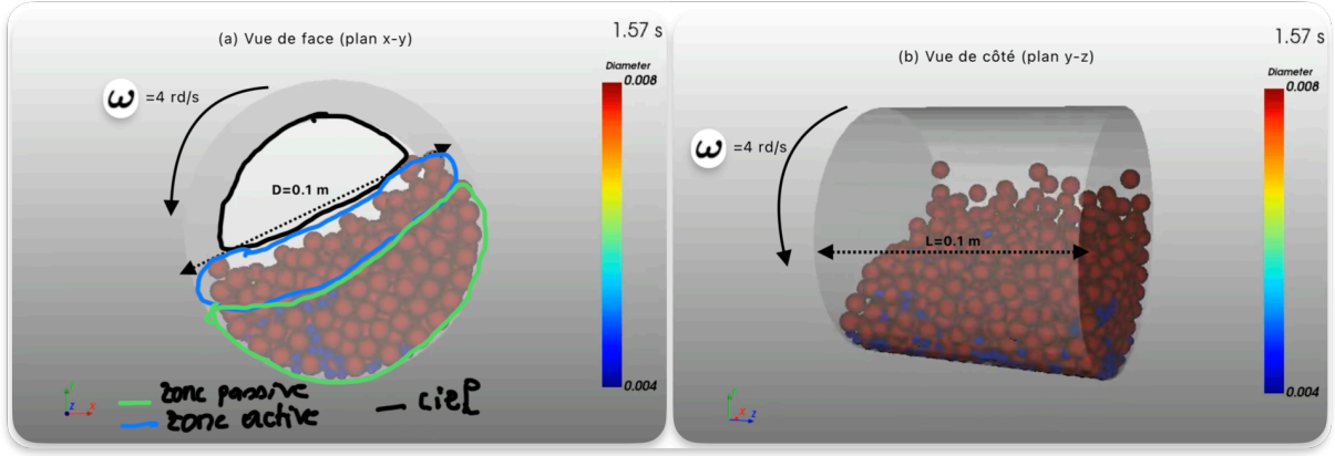
FIGURE 1 – Géométrie du tambour tournant : (a) vue de face avec le lit granulaire incliné, (b) vue de côté . Le tambour de dimensions caractéristiques D = 2R = 0.1m et L = 0.1m tourne à \omega = 4 \text{ rad/s} autour de l'axe z .
