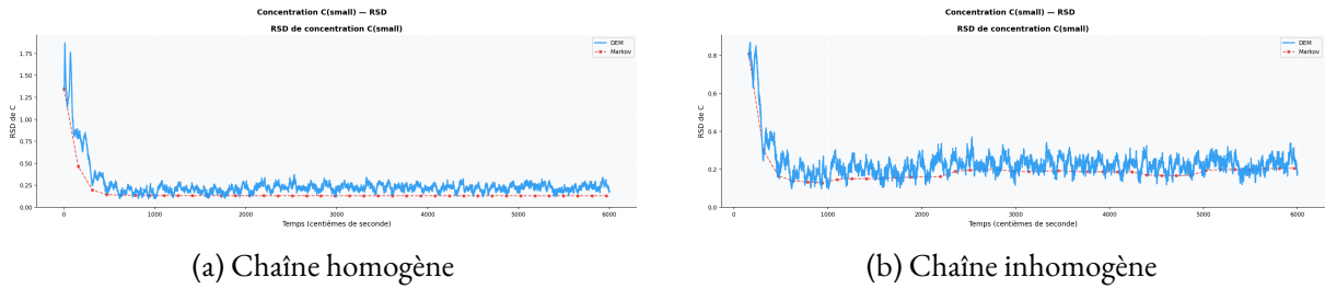
FIGURE 24 – RSD de la concentration en petites particules : DEM vs. Markov homogène et inhomogène (découpage physique).
