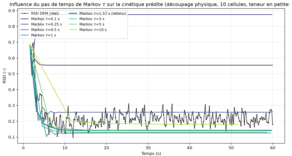
FIGURE 26 – Influence du pas de temps de Markov \tau sur la cinétique de mélange prédite, calculée sur les données DEM (découpage physique, 10 cellules) : RSD DEM de la teneur en petites particules (noir) et prédictions markoviennes homogènes pour \tau de 0,1 s à 10 s. La courbe épaisse correspond à la valeur retenue \tau = 1,57 \text{ s} .
