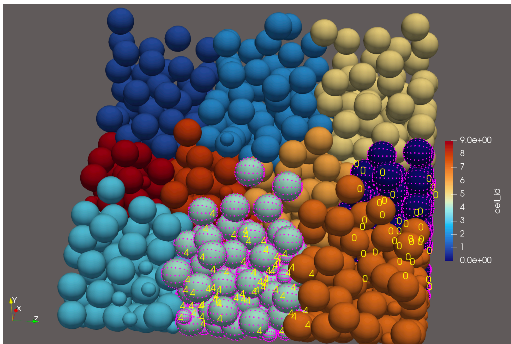
FIGURE 12 – Mélangeur discrétisé en cours de simulation : chaque couleur identifie une cellule ( cell_id ) du découpage. Les cellules du bas, en zone passive, sont nettement plus peuplées que celles de la surface; les petites particules (mises en évidence) se concentrent dans certaines cellules, signature de la ségrégation.
