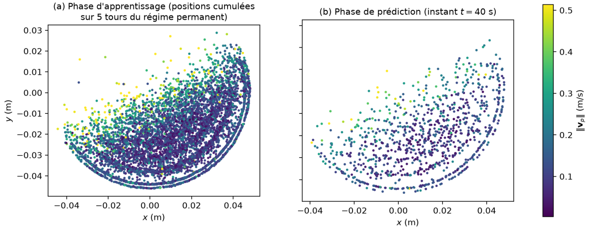
FIGURE II – Espace des caractéristiques du découpage physique : positions des 1030 particules colorées par la norme de leur vitesse, (a) cumulées sur la fenêtre d'apprentissage (cinq tours du régime permanent) et (b) à un instant de la phase de prédiction. La zone active de surface (vitesses élevées, teintes claires) se distingue nettement de la zone passive du cœur du lit (vitesses faibles, teintes sombres) : c'est ce contraste que la quatrième caractéristique \|\mathbf{v}_p\| permet de séparer.
