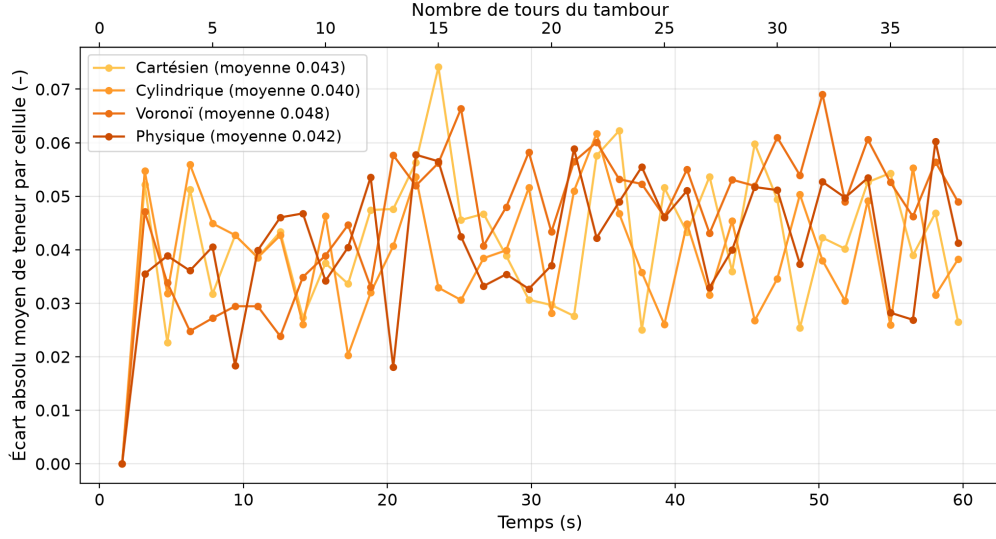
FIGURE 23 – Approche globale sur les courbes de teneur : écart absolu moyen de teneur par cellule entre la prédiction markovienne homogène et la référence DEM, pour les quatre méthodes de découpage à nombre de cellules identique (10 cellules, configuration nlt = 2 , start = 1,57 s, step = \tau = 1,57 s, dt = 8 pas).
