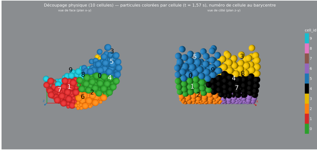
FIGURE 20 – Découpage physique (10 cellules) à t = 1,57 s.
