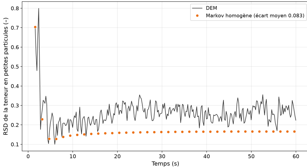
FIGURE 19 – RSD de la concentration en petites particules, découpage de Voronoï, 10 cellules, configuration nlt = 2 , start = 1,57 s, step = \tau = 1,57 s, dt = 8 pas.
