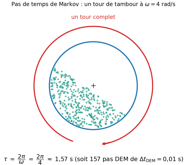
FIGURE 26 – Correspondance entre le pas de temps de Markov \tau et un tour complet du tambour tournant à \omega = 4 rad/s : \tau = 2\pi/\omega \approx 1,57 \text{ s} = 157 pas DEM.
