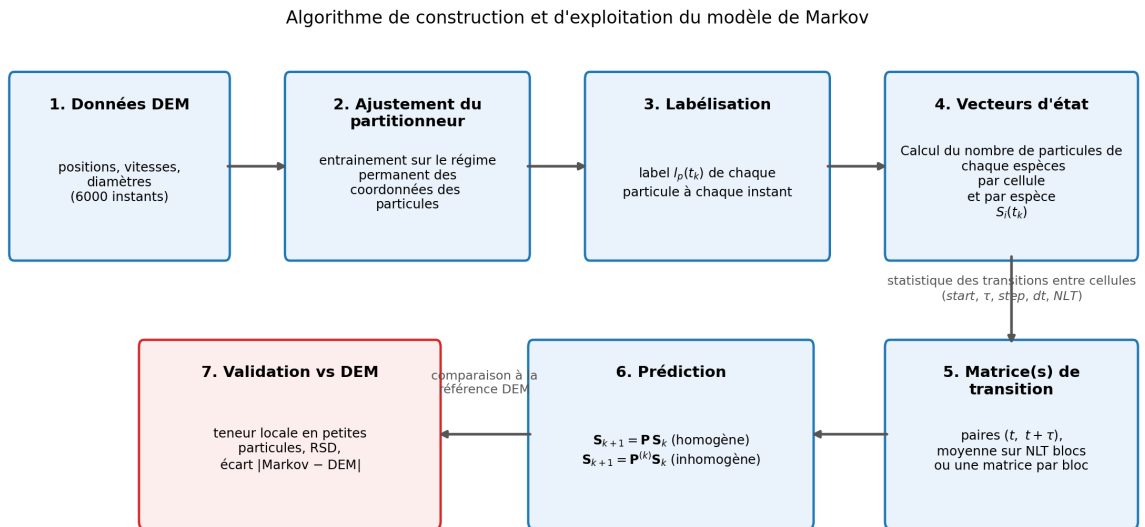
FIGURE 6 – Algorithme de construction et d'exploitation du modèle de Markov : les données DEM servent d'abord à ajuster la méthode de maillage sur le régime permanent, puis à labéliser chaque particule à chaque instant; les vecteurs d'état de comptage qui en découlent alimentent l'apprentissage de la ou des matrices de transition, la prédiction, et enfin la validation par confrontation à la référence DEM.
