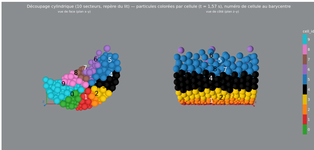
FIGURE 14 – Découpage cylindrique (10 secteurs angulaires dans le repère du lit)
