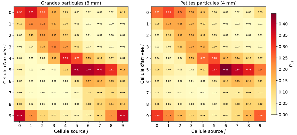
FIGURE 15 – Matrices de transition du découpage cylindrique (10 secteurs angulaires dans le repère du lit; configuration : nlt = 2 , start = 1,57 s, step = \tau = 1,57 s, dt = 8 pas),
