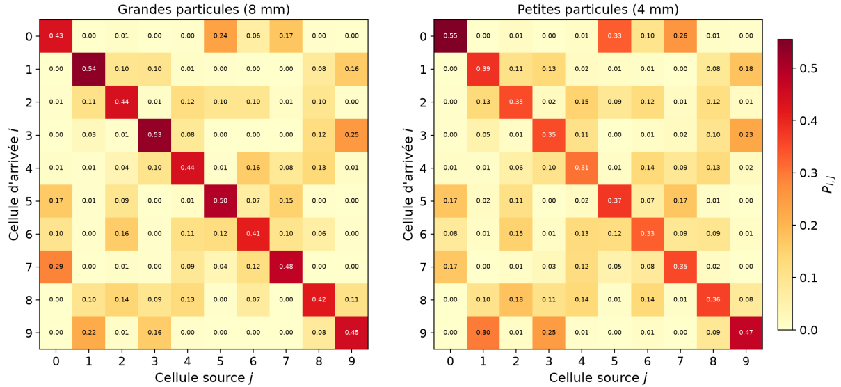
FIGURE 17 – Matrices de transition du découpage de Voronoï (10 cellules, configuration : nlt = 2 , start = 1,57 s, step = \tau = 1,57 s, dt = 8 pas),
