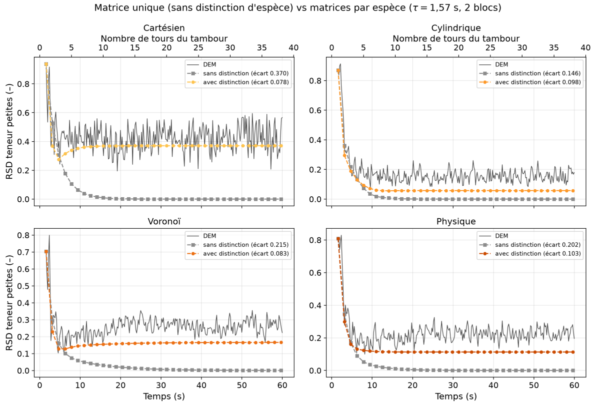
FIGURE 34 – Justification des matrices distinctes par espèce : RSD DEM de la teneur en petites particules vs prédictions markoviennes construites sans distinction d'espèce (matrice unique, gris) et avec distinction (matrices par espèce, couleur), pour les quatre méthodes de découpage (configuration : nlt = 2 , start = 1,57 s, step = \tau = 1,57 s, dt = 8 pas).
