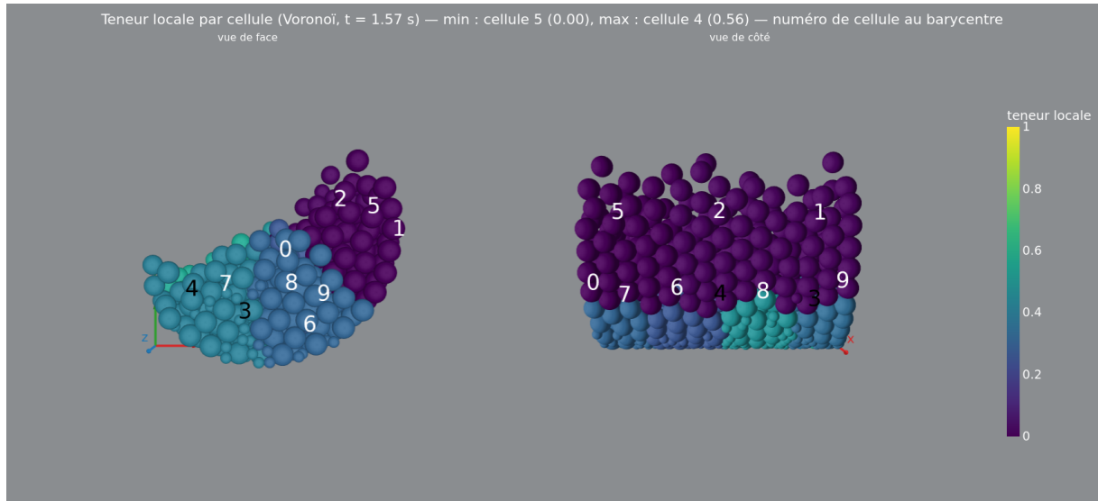
FIGURE 21 – Mélangeur discrétisé en cellules de Voronoï sur la configuration de référence nlt = 2 , start = 1,57 s, step = \tau = 1,57 s, dt = 8 pas
