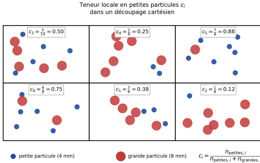
FIGURE 40 – Illustration de la teneur locale en petites particules c_i dans un découpage cartésien : rapport du nombre de petites particules (bleu) au nombre total de particules de la cellule. Les écarts de teneur entre cellules signent la ségrégation.
