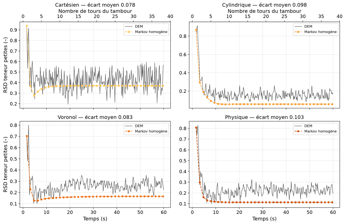
FIGURE 27 – Influence de la méthode de découpage sur la prédiction : RSD DEM vs prédiction markovienne homogène pour les quatre méthodes, à nombre de cellules identique (10 cellules) et à configuration identique ( nlt = 2 , start = 1,57 s, step = \tau = 1,57 s, dt = 8 pas).
