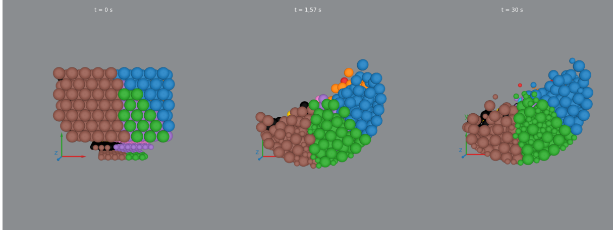
FIGURE 5 – Mélangeur discrétisé (découpage de Voronoï, 10 cellules) aux mêmes instants : chaque particule porte la couleur de la cellule qui la contient; la dynamique particulière est agrégée à l'échelle de ces cellules.
