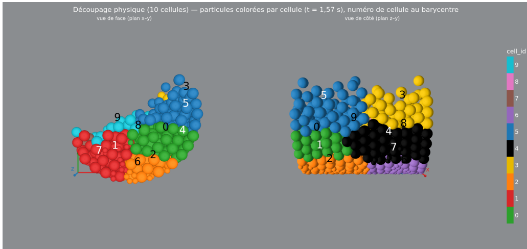
FIGURE 24 – Découpage physique (10 cellules) à t = 1,57 s.
