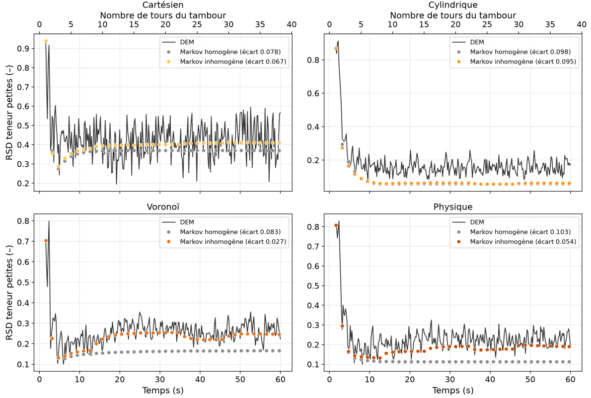
FIGURE 30 – RSD de la teneur en petites particules : référence DEM (trait continu), prédictions homogène (gris) et inhomogène (couleur) pour les quatre méthodes, 10 cellules chacune ( start = 1,57 s, \tau = 1,57 s, dt = 8 pas; chaîne inhomogène : blocs espacés de 7 tours, soit 5 matrices).
