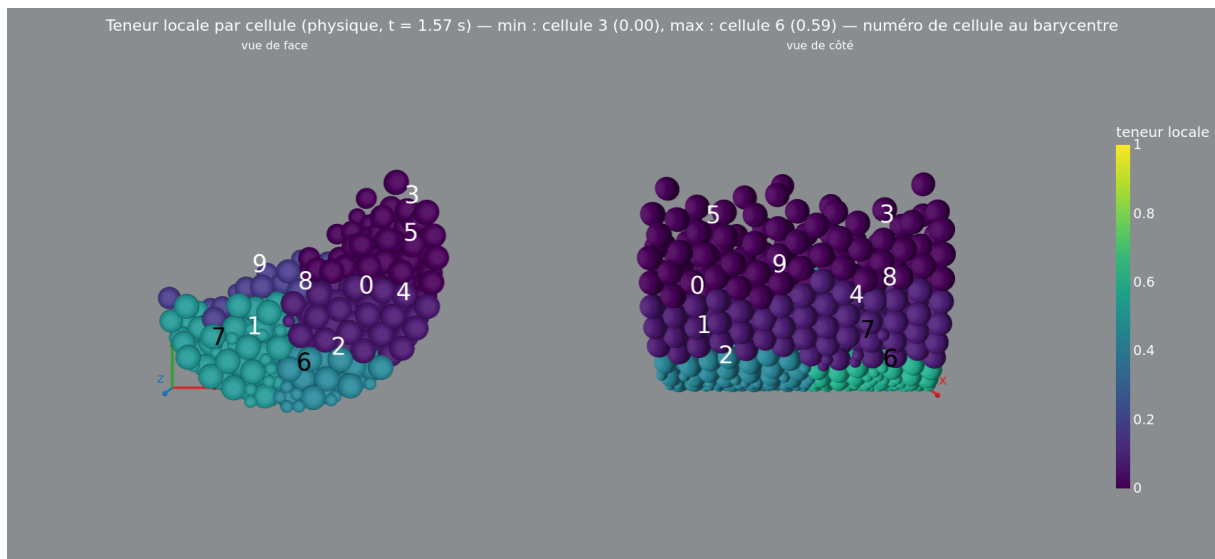
FIGURE 26 – Mélangeur discrétisé par le découpage physique coloré par la teneur locale de chaque cellule à t = 1,57 s, vues de face et de côté; numéro de cellule au barycentre (configuration : nlt = 2 , start = 1,57 s, step = \tau = 1,57 s, dt = 8 pas).
