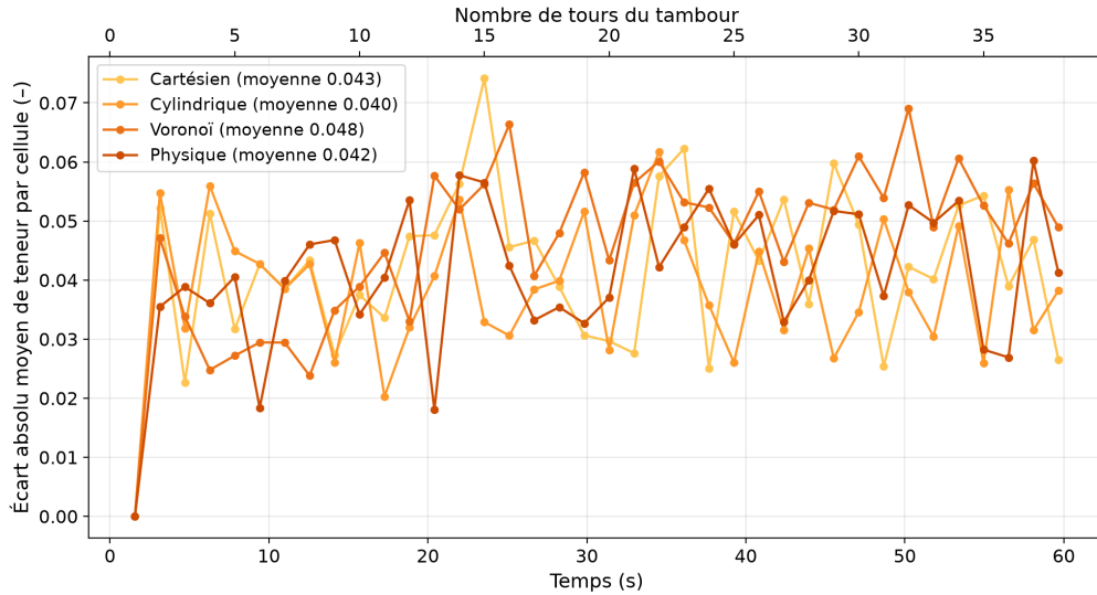
FIGURE 28 – Approche globale sur les courbes de teneur : écart absolu moyen de teneur par cellule entre la prédiction markovienne homogène et la référence DEM, pour les quatre méthodes de découpage à nombre de cellules identique (10 cellules, configuration nlt = 2 , start = 1,57 \text{ s} , step = \tau = 1,57 \text{ s} , dt = 8 \text{ pas} ).
