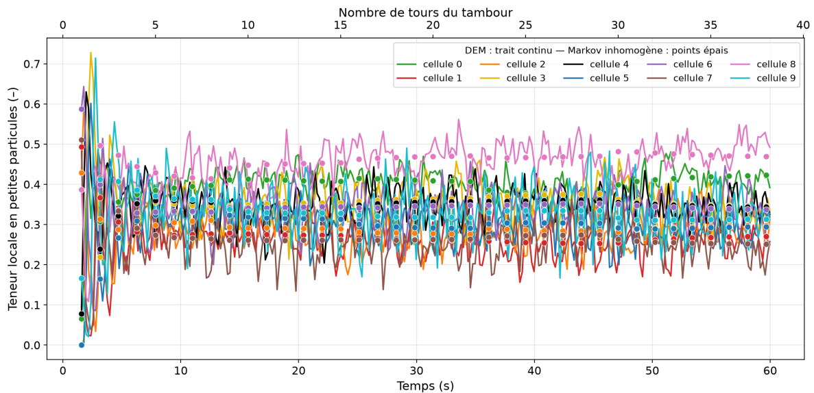
FIGURE 29 – Teneur locale en petites particules par cellule : référence DEM (trait continu) et prédiction de la chaîne inhomogène (marqueurs épais), découpage physique, 10 cellules ( start = 1,57\text{ s} , \tau = 1,57\text{ s} , dt = 8\text{ pas} ; blocs espacés de 7 tours, soit 5 matrices).
