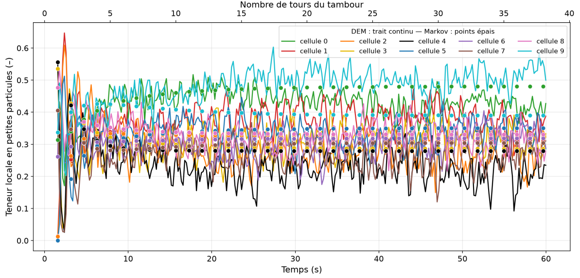
FIGURE 20 – Teneur locale en petites particules par cellule Voronoï, 10 cellules, configuration nlt = 2 , start = 1,57 s, step = \tau = 1,57 s, dt = 8 pas.
