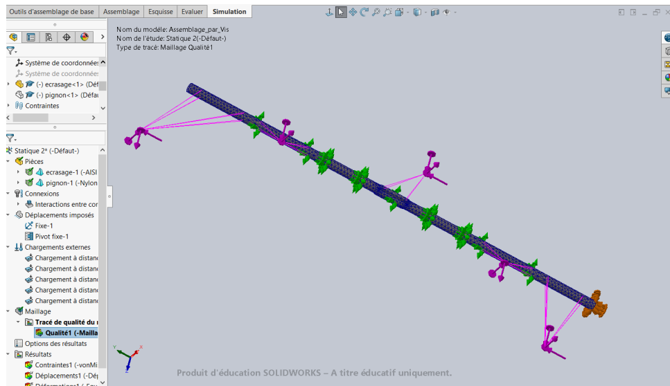
FIGURE 9 – Application des efforts et les chargements sur l'axe
