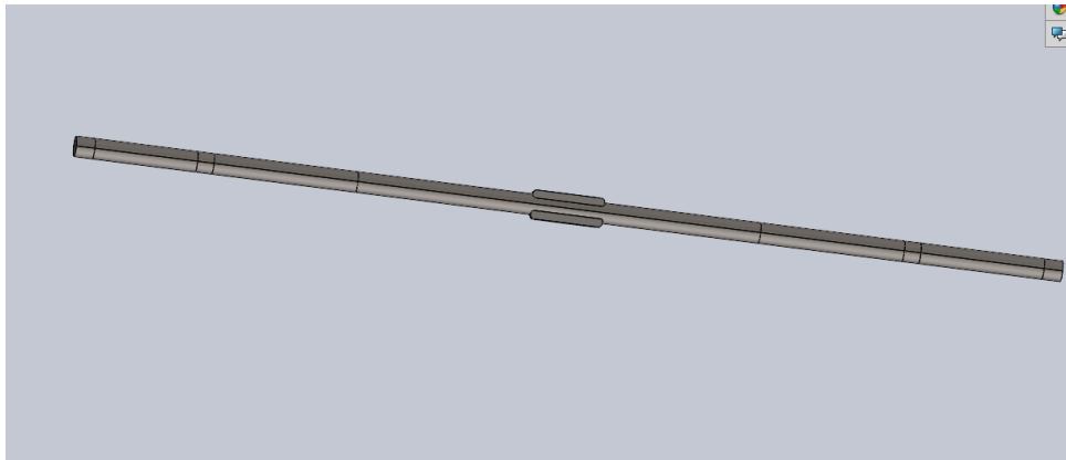
FIGURE 7 – Modélisation de l'axe arrière et répartition des liaisons
