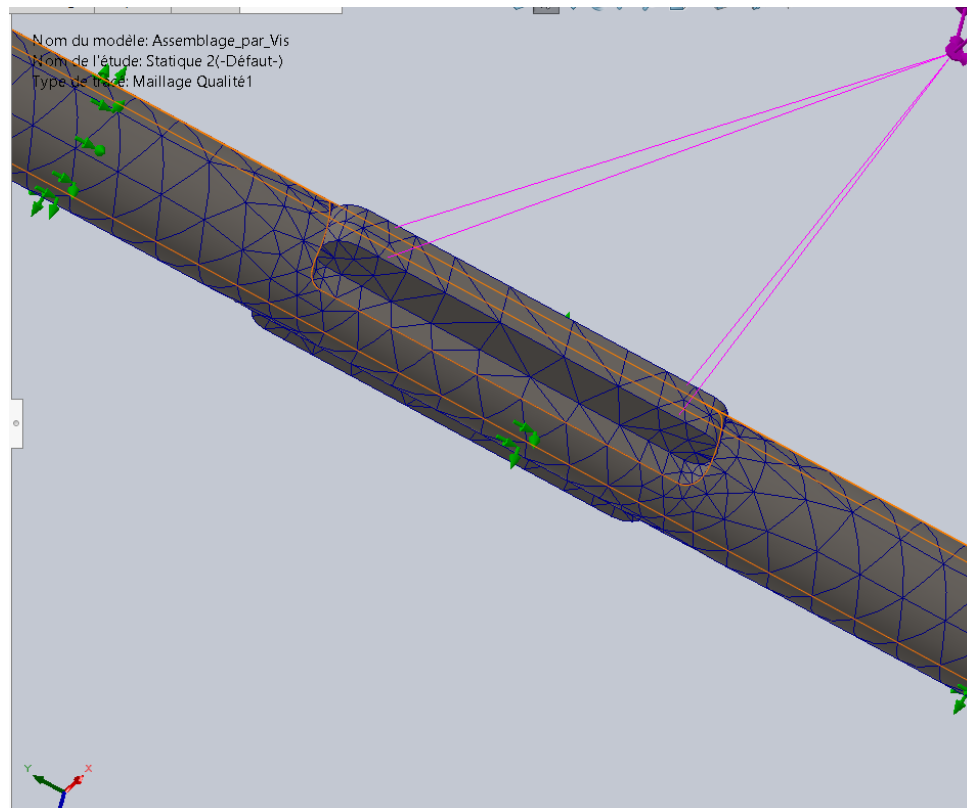
FIGURE 10 – Modèle de maillage
