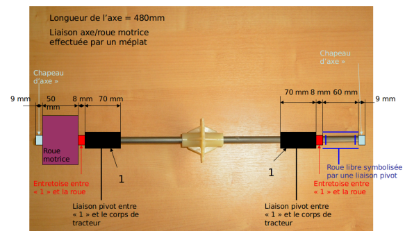
FIGURE 5 – Schéma des liaisons de l'axe arrière avec la fixation du pignon
