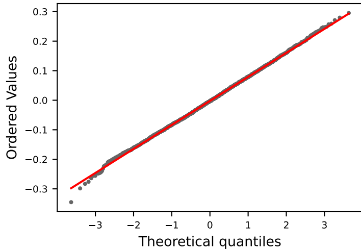
Normal Q-Q
